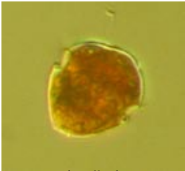
Peridiniella danica
