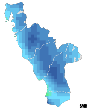
Beräknat 2069-2098
