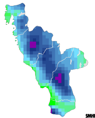
Beräknat 2069-2098
