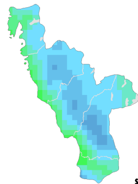
Beräknat 2069-2098
