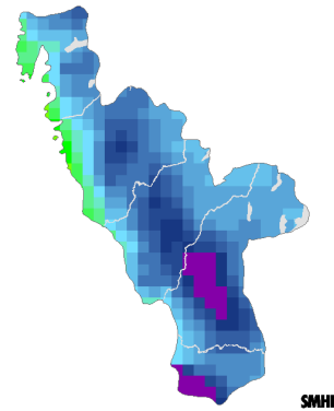
Beräknat 2069-2098
