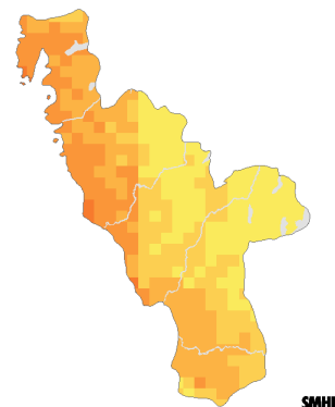
Beräknat 2021-2050
