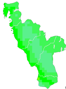
Beräknat 2069-2098
