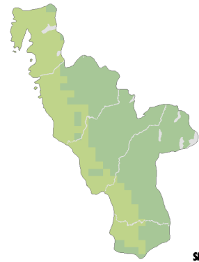
Beräknat 2069-2098
