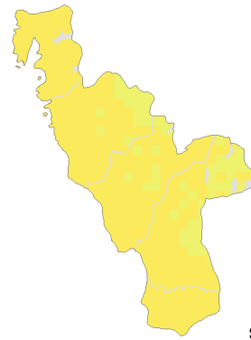
Beräknat 2069-2098
