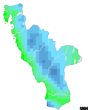
Beräknat 2069-2098
