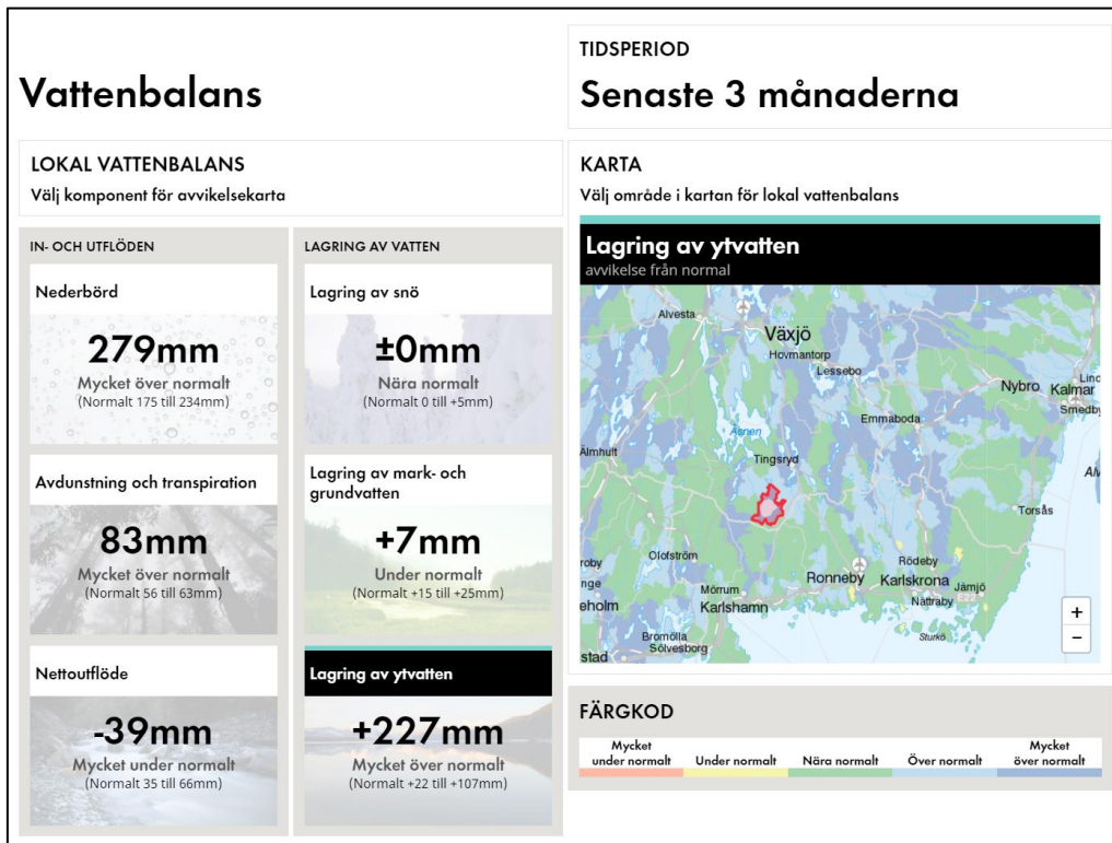
Figur. SMHIs nya tjänst Vattenbalans som presenterar vattenbalansberäkningar för ett lokalt område. I detta exempel har området kring sjön Mien valts. Kartan visar hur de senaste tre månadernas förändring av ytvattenlagret avviker från normala värden. I Mien är förändringen mycket över normalt (+227 mm jämfört med normalt +22 till +107 mm), men notera att dessa siffror inte visar ytvattenlagrets storlek, d.v.s. vattenståndet i Mien. Källa: SMHI Vattenwebb
