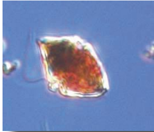
Heterocapsa triquetra
