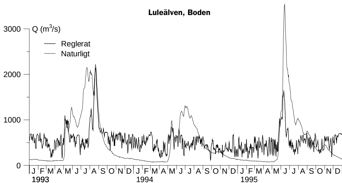
Figur 4. Jämförelse mellan den reglerade vattenföringen i Luleälven, vid Boden, och en rekonstruktion av de förhållandena som rått om älven inte varit utbyggd (dygnsmedelvärden).
