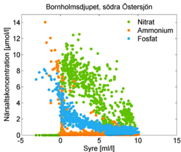
Koncentrationen av närsalter påverkas i hög grad av syreförhållandena. Figuren visar relationen mellan oorganiska närsalter (nitrat, ammonium och fosfat) och syre i södra Östersjön (Bornholmsdjupet) för hela vattenmassan under perioden 2001 – 2010.
