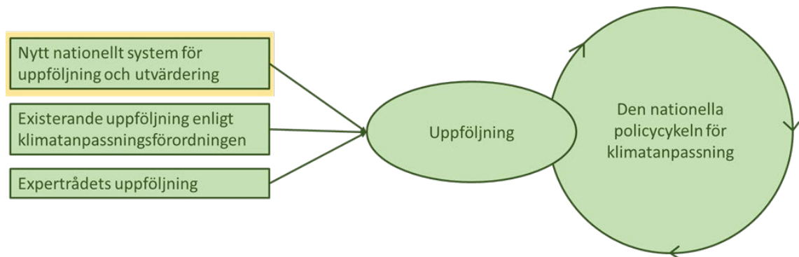
Figur 1: Förslagens struktur
