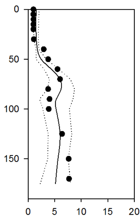
DIN μmol/l
