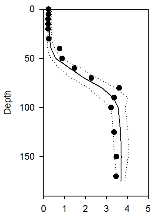
PO 4 μmol/l
