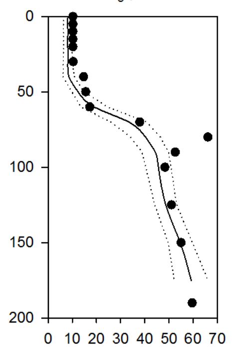
SiO 3 μmol/l
