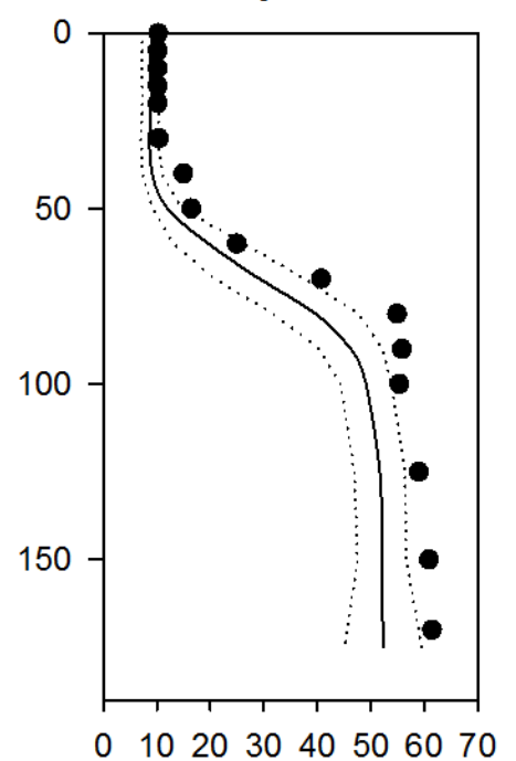
SiO 3 μmol/l
