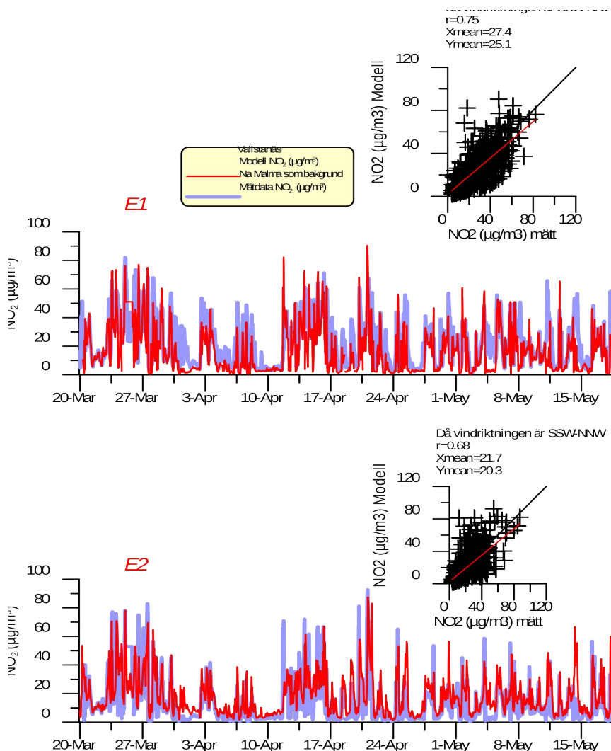
Figur 3.6.2.1 Jämförelse mellan beräknade och uppmätta halter av NO 2 (mg/m 3 ) vid E4:an norr om Stockholm (Vallstanäs).
