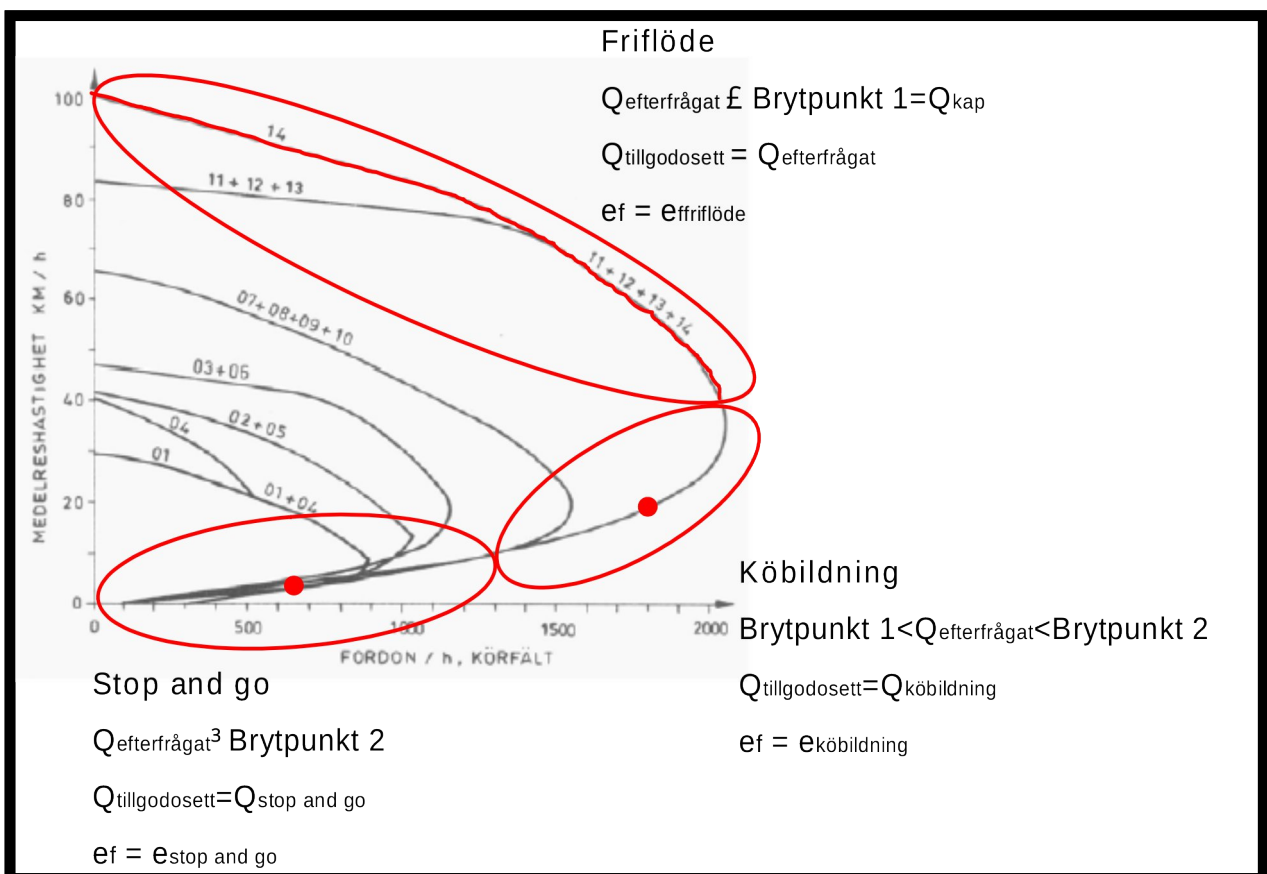
Figur 3.1.1.3 Indelning av emissionssambanden görs i tre klasser: friflöde, köbildning och stop and go.
