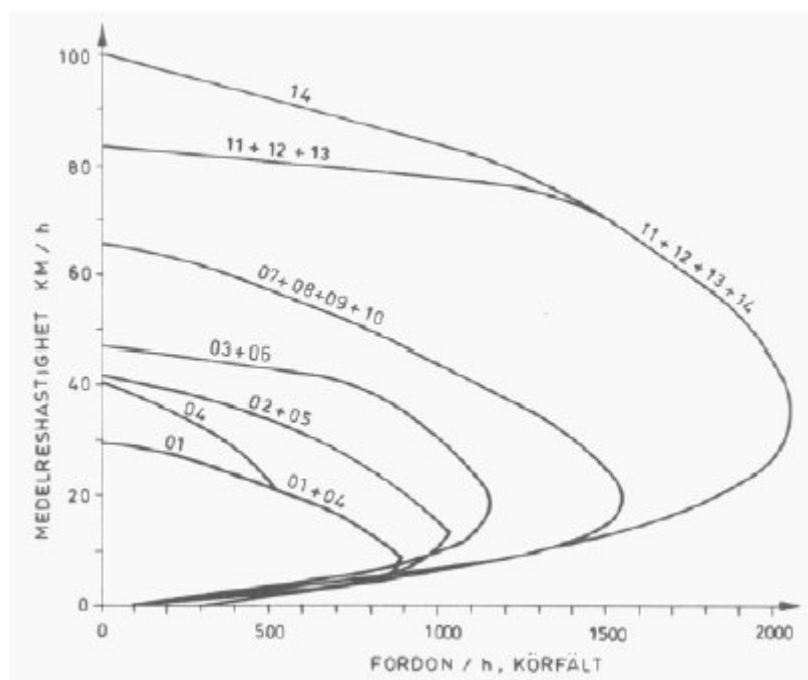
Figur 3.1.1.2 TU71-sambanden emellan trafikflöde och medelres hastighet (inklusive korsning).
