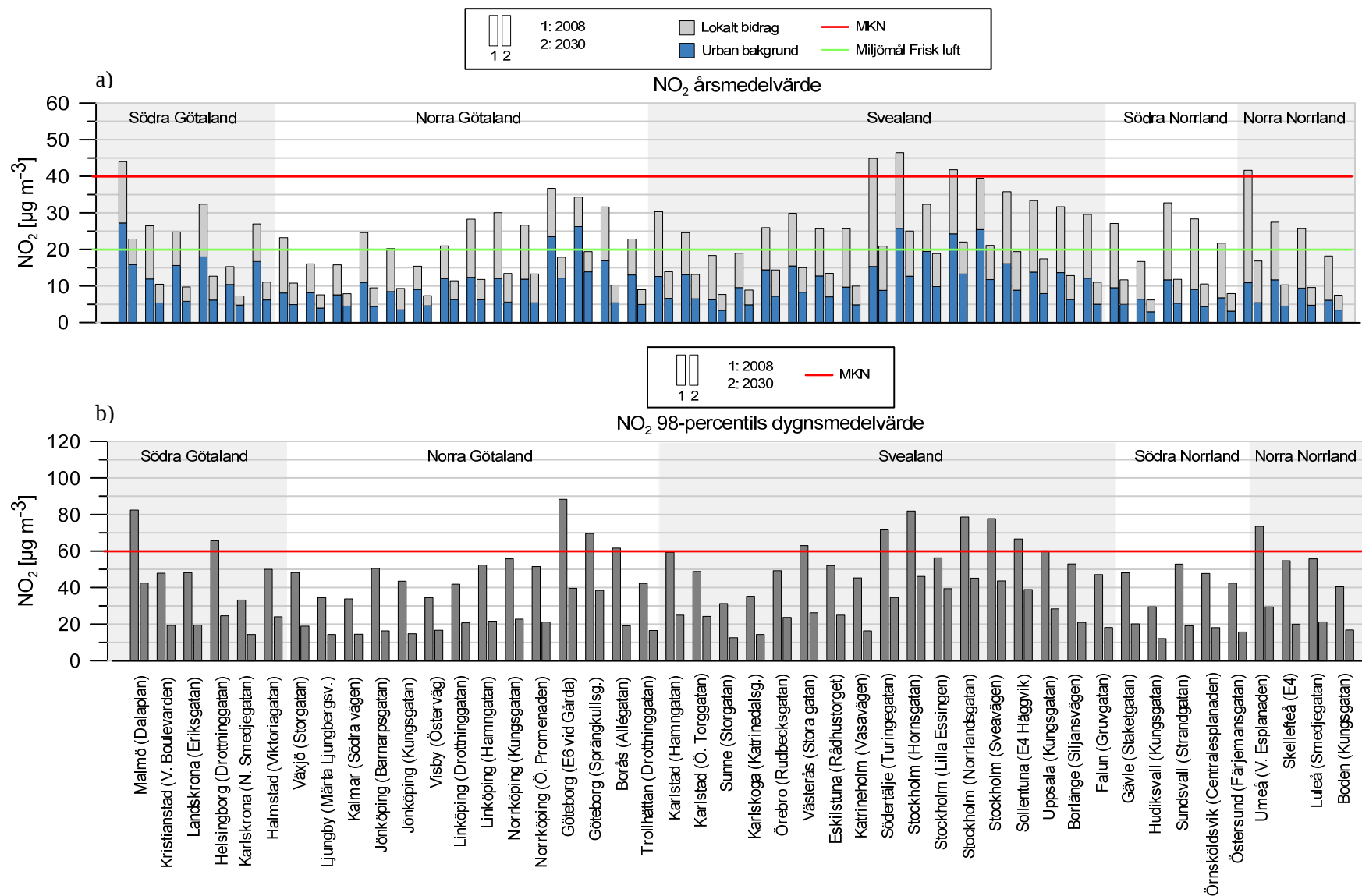
Figur 20. NO 2 – Figurtext, se nästa sida.
