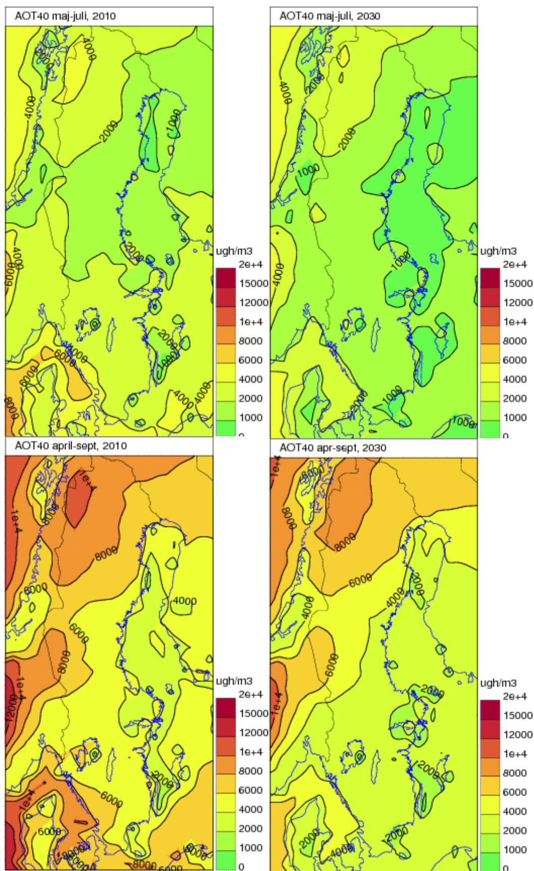
Figur 10. AOT40 år 2010 till vänster, och år 2030 till höger, för perioden maj till juli. Beräkningarna representerar ett medel baserat på tre meteorologiska år (2007-2009). Enheten är µgh/m³.
