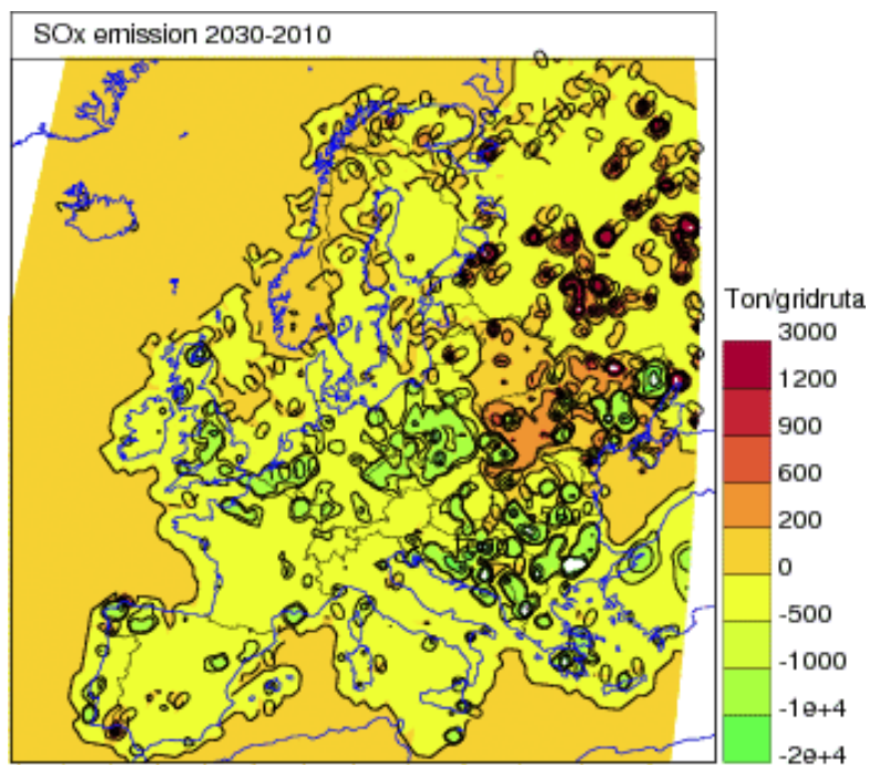
Figur 1. Skillnad i antropogena emissioner av svavel för åren 2010 och 2030. Emissionerna visas som totala emissioner i ton per gridruta (44 x 44 km).
