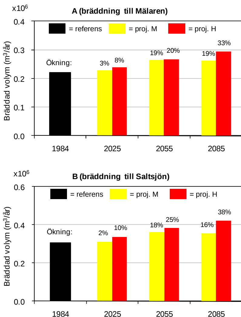
Figur 22. Förändring i bräddad volym till Mälaren (A) och Saltsjön (B) under helåret.
