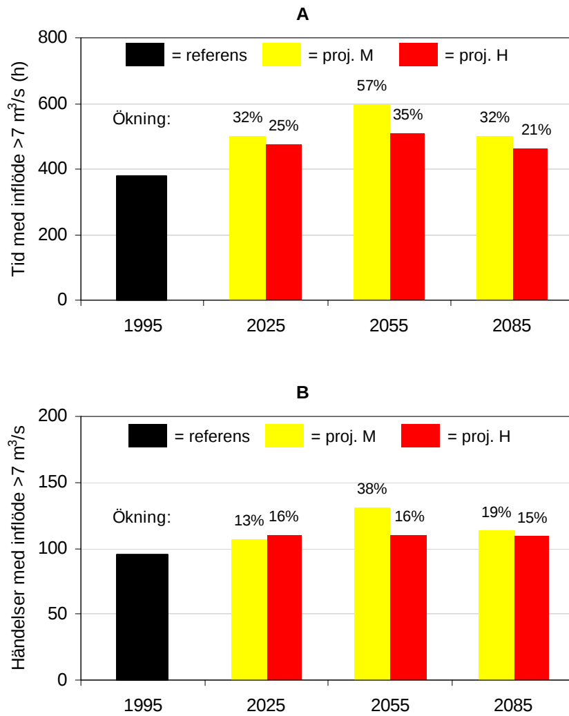
Figur 27. Andel av tid med inflöde >7 m 3 /s (A) och antal regnhändelser med inflöde >7 m 3 /s (B) till Henriksdal.
