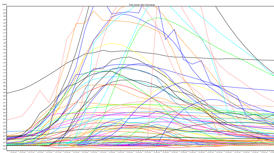
Figur 1: Bräddflöden vid ett 10 års regn.
