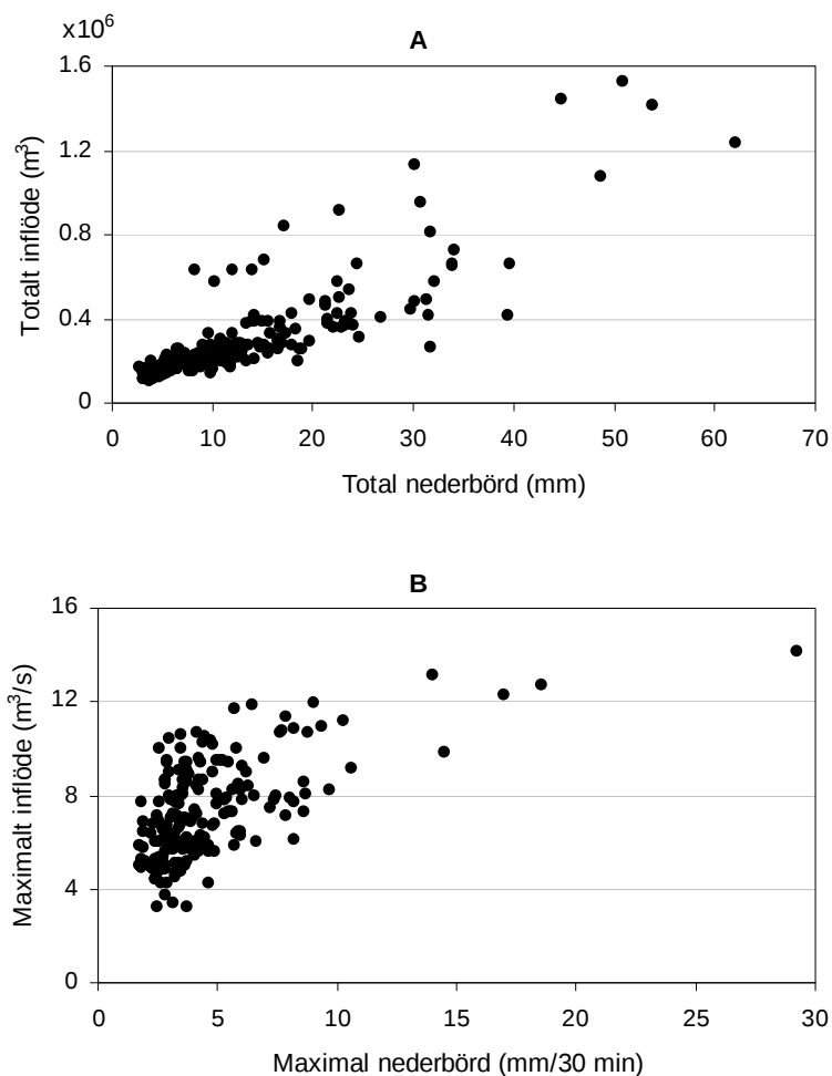
Figur 7. Totalt inflöde som funktion av total nederbörd (A) och maximalt inflöde som funktion av maximal 30-min nederbörd (B) för de utvalda regnhändelserna.
