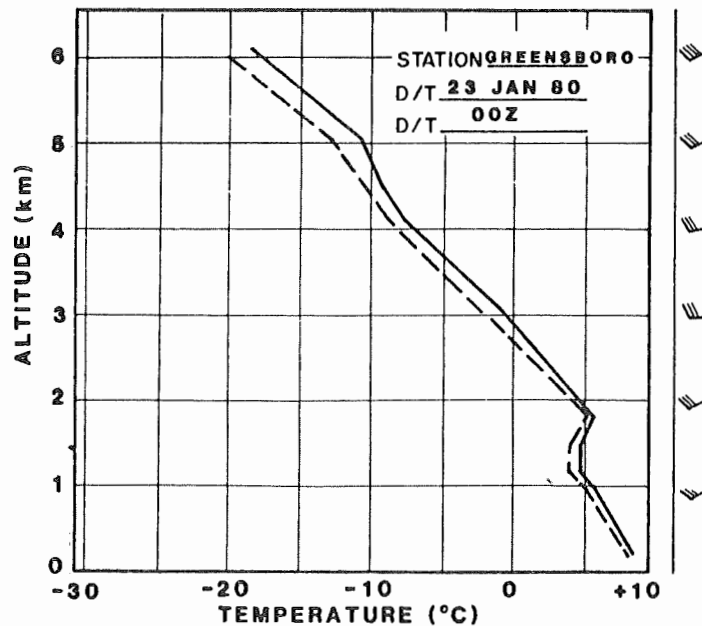
Fig 5c: Sondering genom en varmfront som gav ihållande måttligt-kraftigt regn, men endast SPORADISKT LÄTT ISBILDNING. Droppspektrum var smalt med stora droppar, diameter i regel över 400 \mu m. Att isbildningen trots detta nästan uteblev kan förklaras dels av att få underkyllda droppar fanns (de flesta var frusna tills de nådde under 0°C-isotermen), dels av att vatteninnehållet i nederbörd är relativt litet (400 \mu m är nederbördsstorlek).
