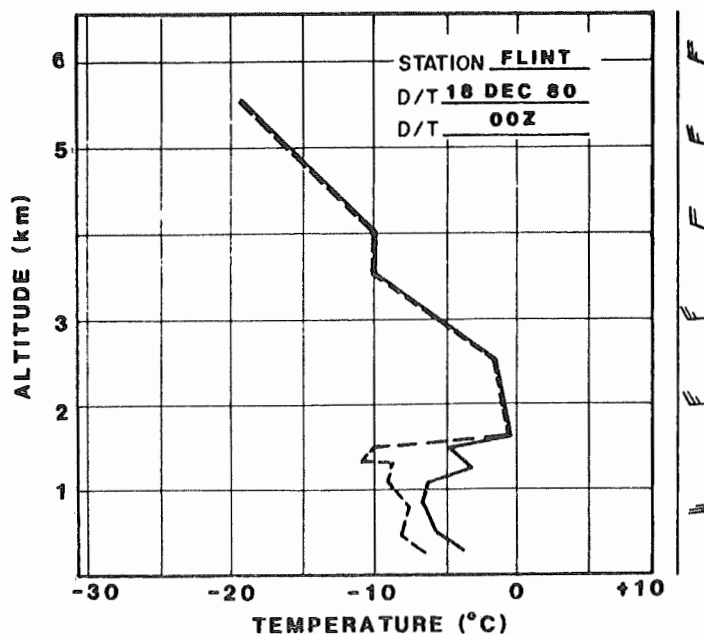
Fig 5d: Sondering genom en varmfront som gav intermittent snöblandat regn och MÄTTLIG ISBILDNING. Droppspektrum var bredare än i Fig 5c och det fanns gott om underkyllda molndroppar.
