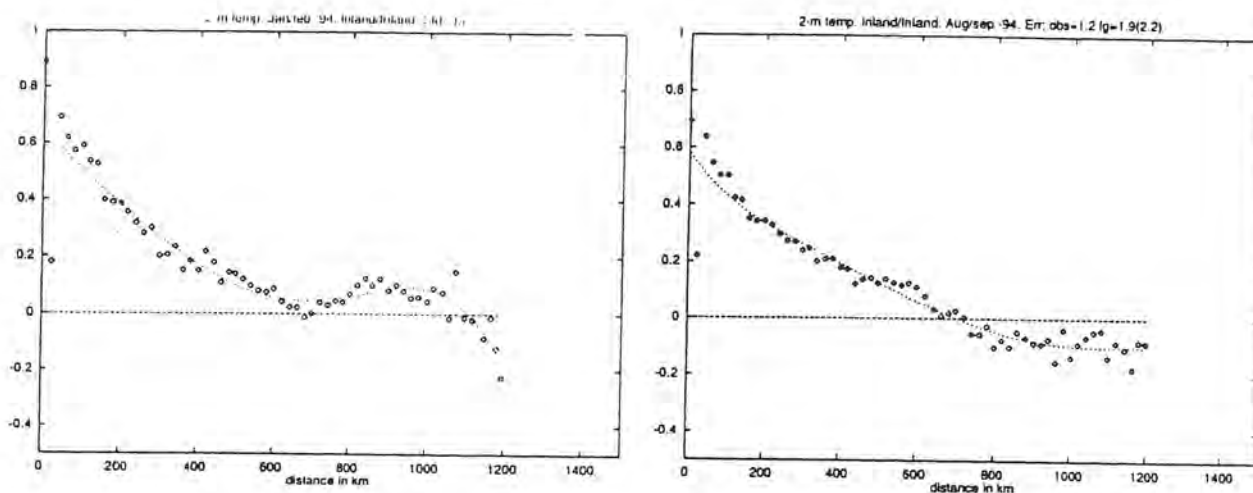
Figur 28 a) Korrelationen hos förstagissningsfelet som funktion av avstånd för inlandsstationer under januari/februari. b) som a men för perioden augusti/september.
