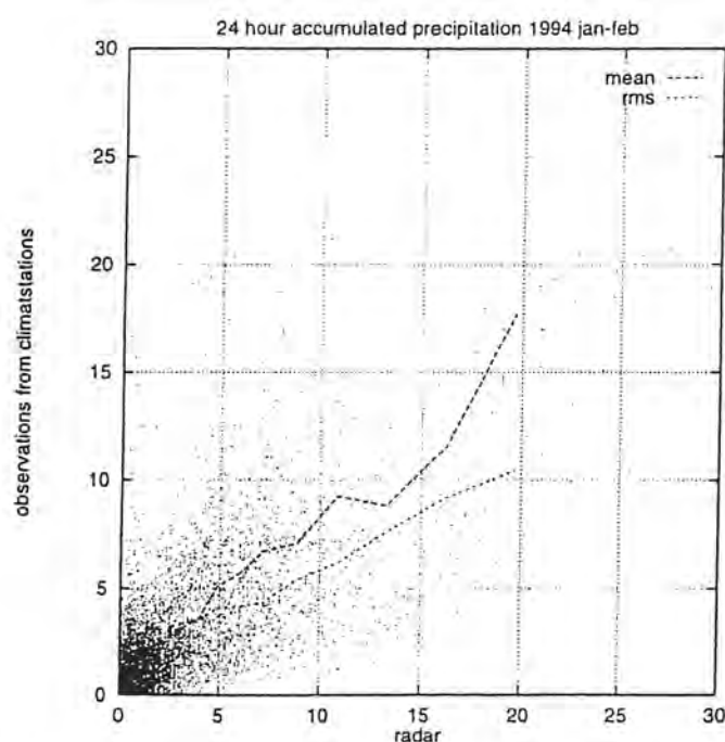
Figur 8. De från radar ackumulerade nederbördsmängderna plottade (x-axeln) mot klimatstationsobservationerna (y-axeln). Den övre kurvan visar medelvärde för klimatstationer vid olika radarnederbörd och den undre rms-avvikelse.
