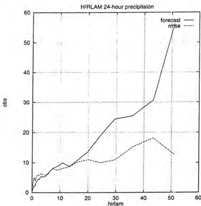
Figur 2. Av Hirlam prognoserad 24-timmars nederbörd (x-axeln) mot observerad (y-axeln).
