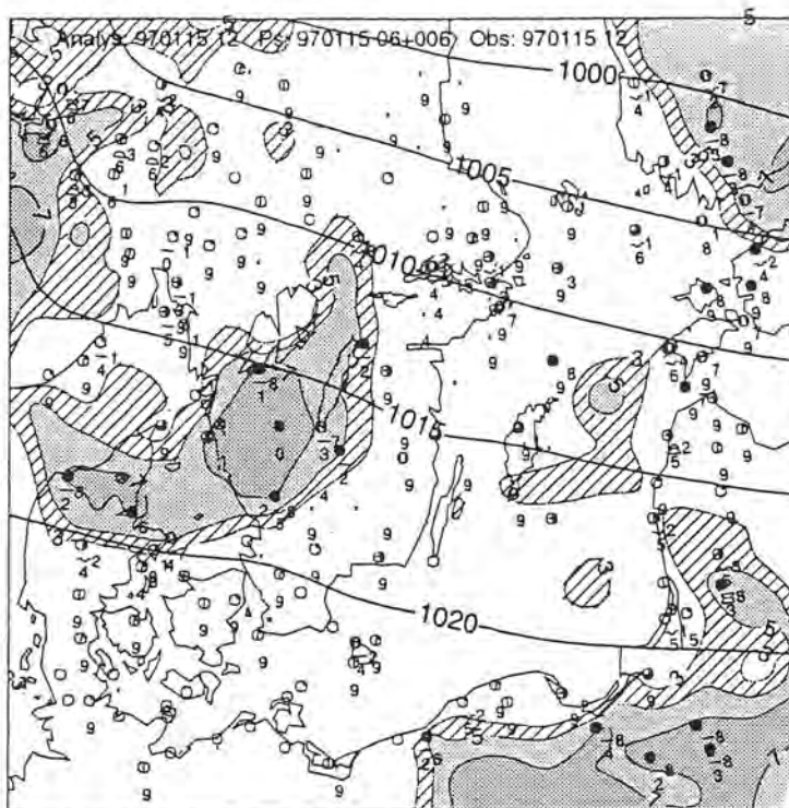
Figur 58. Analys av mängd låga moln gällande den 15 januari 1997 klockan 12 UTC. Sträckat 3-5, ljus skuggat 5-7 och mörkt skuggat 7-8/8 moln. Analysen är baserad på synop, metar, automatstaionsdata och dessutom klassade NOAA-data. Till första gissningen har data från Hirlam använts.
