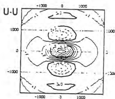
Figur 37: Motsvarande figur 36 men för fria atmosfären enligt (Lönnberg och Shaw 1987)
