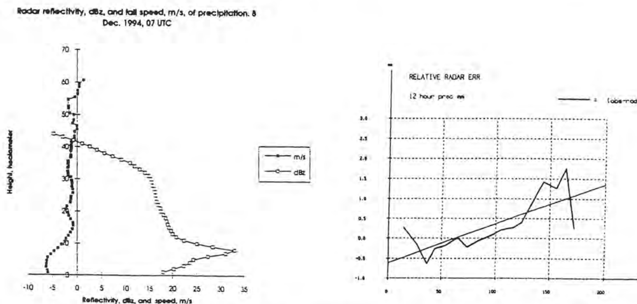
Figur 4. a) Radarprofil från dec. 94. Ofyllda fyrkanter, reflektivitet i dbz och fyllda fallhastighet i m/s (efter Tage Anderson SMHI). b) Relativa radarfelet (obs-rad)/rad som funktion av avstånd från radarn. Nära radarn sker en viss överskattning av nederbörden medan den på lägre avstånd underskattas. Figuren visar fall då radarn under 12 timmar gav mellan 1 och 3 mm, dvs fall då radarn inte gav nederbörd har utesluts.
