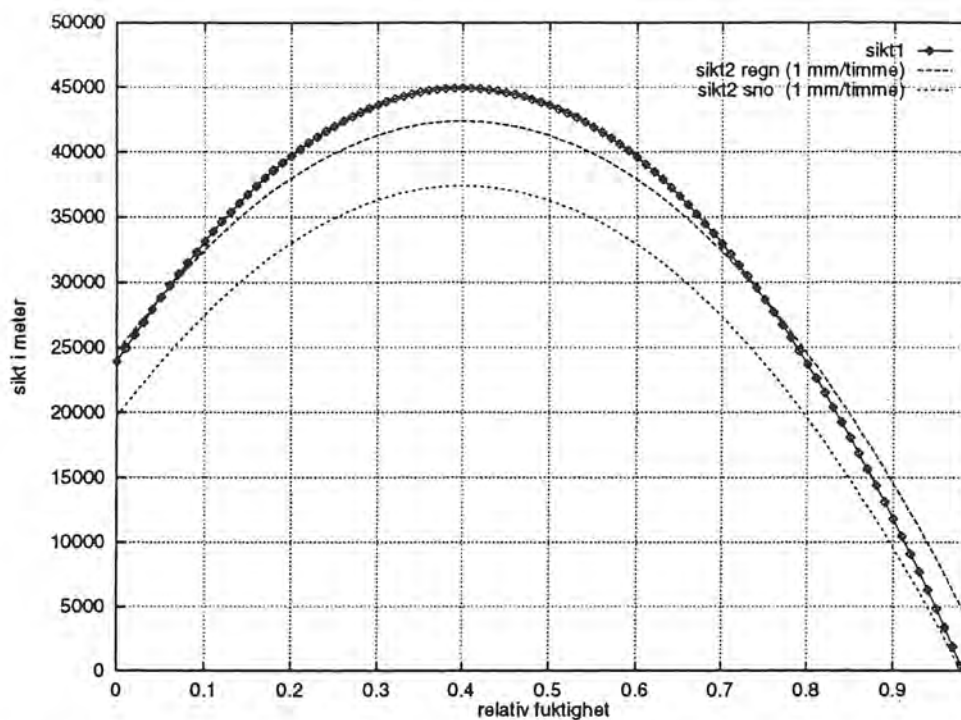
Figur 51. Använda relationer för att från analys av relativ fuktighet och nederbörd skapa ett första gissningsfält för sikt. Kurva sikt1 visar relationen mellan relativ fuktighet och sikt vid uppehåll och kurva sikt2 vid nederbörd (1 mm/timme) i form av regn respektive snöfall.
