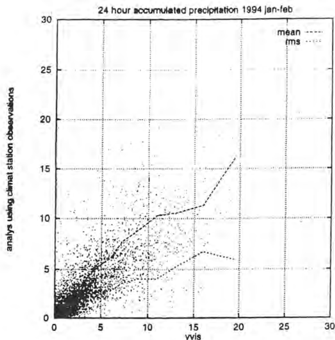
Figur 11. De från VViS beräknade nederbördsmängderna plottade (x-axeln) mot de från analysen av klimatstationsobservationerna interpolerade värdena (y-axeln). Den övre kurvan visar medelvärden och den undre rms-avvikelse.
