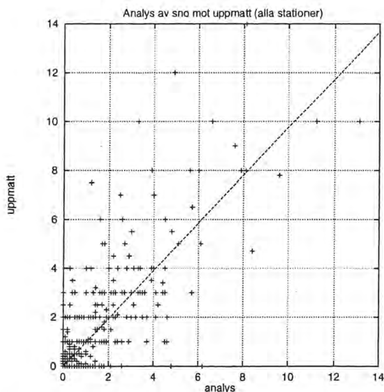
Figur 19. Jämförelse mellan analyserat snödjup och uppmätt. Alla stationer för månaderna januari, februari och mars -96. Analyserna har integrerats att gälla samma tidsupplösning som observationerna.
