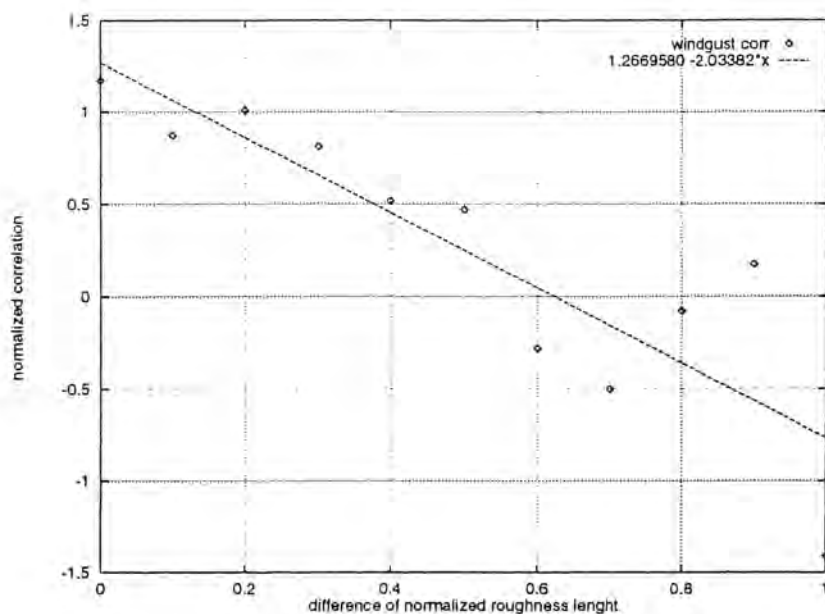
Figur 43. Korrelationerna har först normaliserats med medelvärdet av korrelationen för stationernas horisontella avstånd. Därefter har relativ ändring i korrelation som funktion av skillnad i normaliserad skrovlighet beräknats och plottats i figuren.
