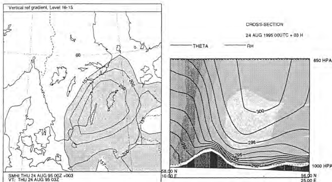
Figur 6. a) Refraktivitetsgradient från Hirlam, modellnivå 15-16. I områden som skuggas kan anomala ekon förväntas förekomma. b) Till höger, ett tvärsnitt från Århus till Riga med potentiell temperatur och fuktighet (mörkt skuggat hög fuktighet).
