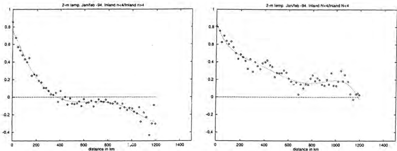
Figur 32. a) Korrelation mellan förstagissningsfel mellan stationer som har mer respektive mindre än 4/8 moln och b) för där båda stationerna har mindre än 4/8 moln.
