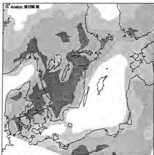
Figur 47 Fukt till sikt (1,4 och 10 km)
