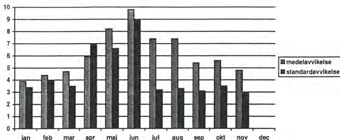
Figur 53. Månadsvisa värden av 2-meterstemperatur minus brightnessstemperatur från METEOSAT vid klart väder och motsvarande standardavvikelse
