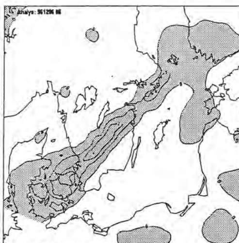
Figur 46. Nederbörd
