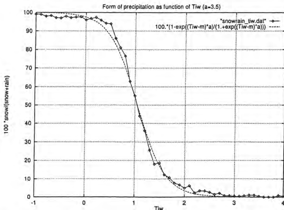
Figur 16. Den från synop observerade frekvensen snö/nederbörd vid olika värden på Tiw. Figuren bygger på synoptiska observationer från perioden januari-mars 1995. Tiw har beräknats från observerad temperatur och daggpunkt. Varje punkt representerar medelvärden av mellan 500 och 1000 observationer.
