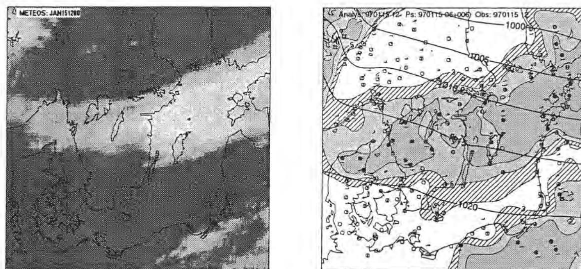
Figur 56. Som ovan men baserad på IR-data från METEOSAT, synop och automatstationsdata. I IR-bilden presenteras höga IR-värd som mörka och låga som ljusa.
