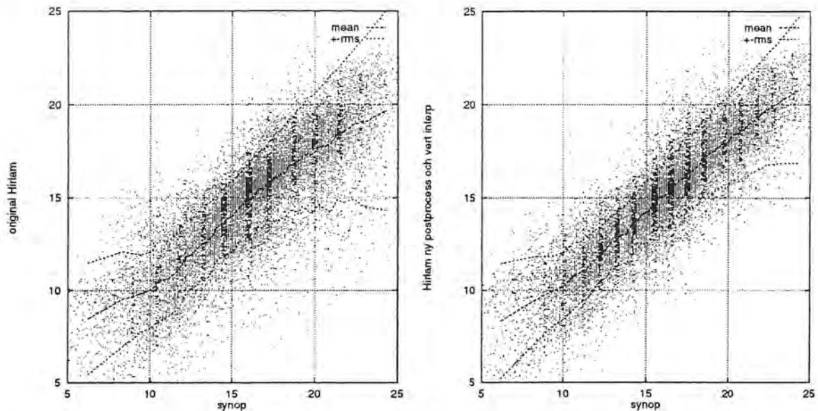
Figur 27 Observerad och beräknad temperatur för perioden 1-10 augusti 1996. Till vänster data från ordinarie postprocessing i Hirlam och till höger med den nya formuleringen och med vertikal interpolation till stationshöjd.
