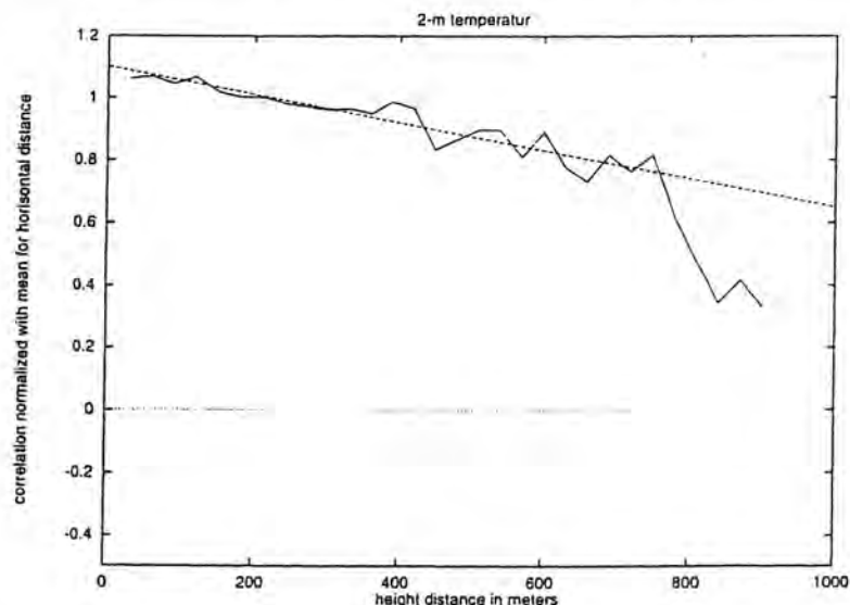
Figur 31. Korrelationen mellan förstagissningsfel hos stationer på olika höjd över havet dividerat med medelvärdet av korrelationen för stationernas horisontella avstånd. Den streckade linjen visar en anpassning till värden för höjdskillnader mindre än 900 meter.
