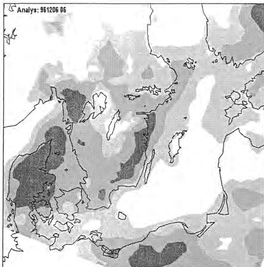
Figur 49. Analyserad sikt, skuggat 1,4,10 km
