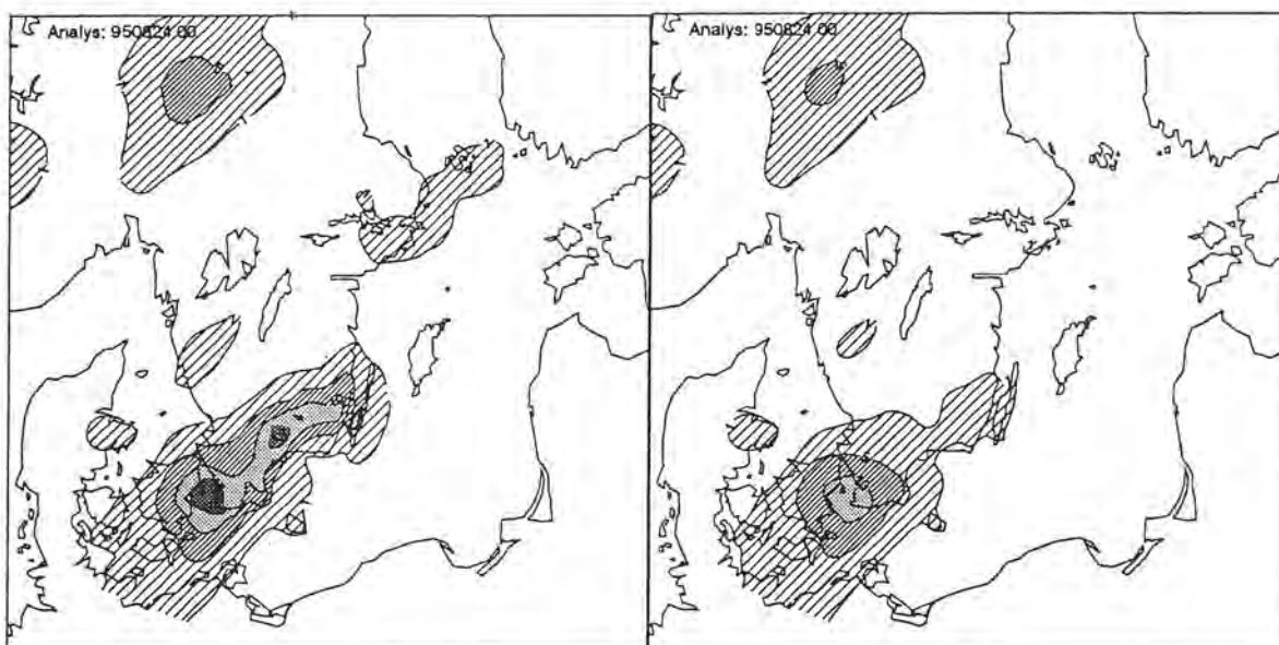
Figur 1. Analys av ackumulerad nederbörd under 3 timmar fram till den 24 augusti kl 00 med synop, radar och första gissning från Hirlam. I a) har en gemensam kvalitetskontroll av alla data använts och i b) har okorrelerade data kontrolleras först och därefter har korrelerade (radar) data kontrollerats mot godkända okorrelerade data. En del felaktig nederbörd finns fortfarande kvar över bl a Blekinge.
