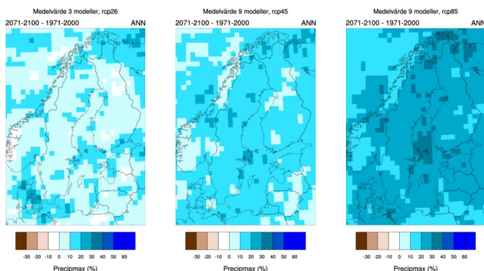
Figur 14. Beräknad förändring av största dygnsnederbörd (procent) för perioden 2071-2100 jämfört med 1971-2000. Kartorna representerar medelvärden av tre (RCP2,6) respektive nio (RCP4,5 och RCP8,5) regionala scenarier där RCA4 drivits av olika globala klimatmodeller.
