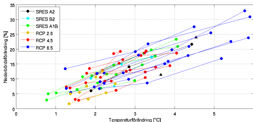
Figur 8. Simulerad förändring i årsmedeltemperatur och nederbörd för Sverige i olika generationer av regionala klimatscenarier från Rossby Centre. För de flesta scenarierna finns tre värden (sammansbundna av en linje) som representerar förändring från 1961-1990 till 2011-2040, 2041-2070 och 2071-2100. För de allra äldsta scenarierna finns bara perioden 2071-2100 med (markerade med trianglar).
