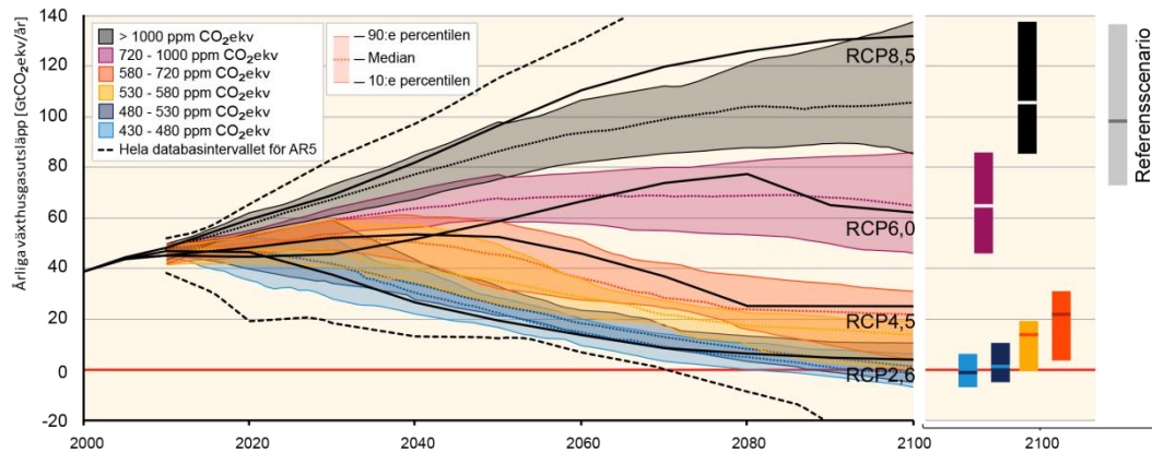
Figur 21 Utvecklingsvägar för globala utsläpp av växthusgaser (GtCO 2 ekv/år) i referens- och utsläppsminskningsscenarier för olika haltnivåer på längre sikt. Översatt från IPCC (2014e).
