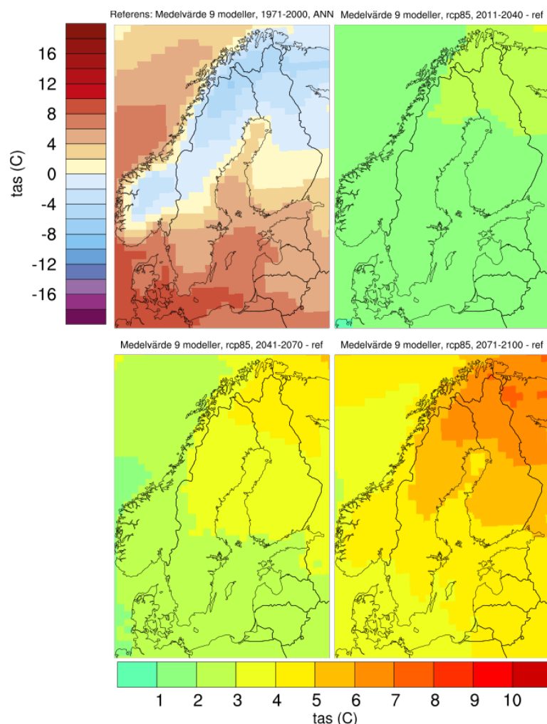
Figur 10: Beräknad årsmedeltemperatur (°C) för 1971-2000 (längst upp till vänster) och förändring i temperatur (°C) för tre framtida perioder 2011-2040; 2041-2070; 2071-2100 för RCP8,5. Samtliga kartor visar ett medelvärde baserat på nio regionala klimatscenarier där olika globala klimatmodeller skalats ner för Europa.
