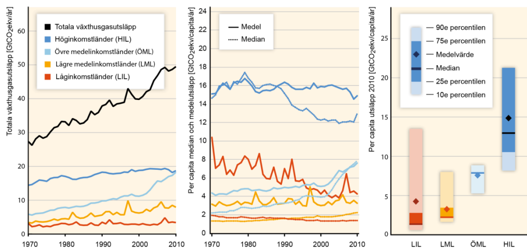
Figur 19 Historisk utveckling av länders växthusgasutsläpp indelat efter inkomstgrupp. Vänster diagram visar totala utsläpp från 1970 till 2010 (miljarder ton CO 2 ekv/år). Mittendiagrammet visar utvecklingen av årliga per capita utsläpp som medel- och medianvärden (ton CO 2 ekv/cap). Höger diagram visar fördelningen av ländernas per capita utsläpp år 2010 inom varje inkomstgrupp (ton CO 2 ekv/cap). Fördelning i inkomstgrupp enligt Världsbankens klassificering. Översatt från IPCC (2014d)
