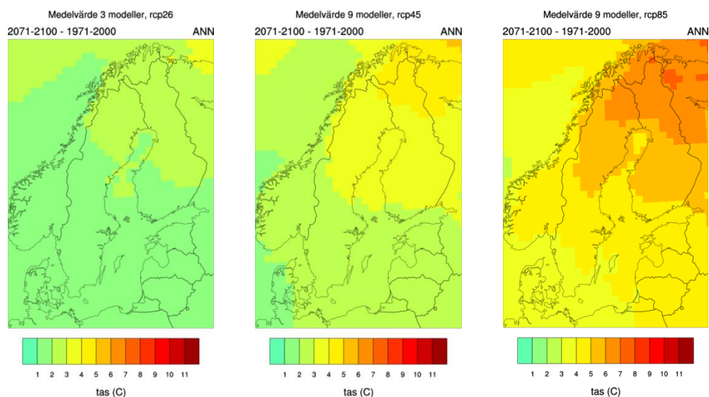
Figur 11: Beräknad förändring av årsmedeltemperaturen (°C) för perioden 2071-2100 jämfört med 1971-2000. Kartorna representerar medelvärden av tre (RCP2,6) respektive nio (RCP4,5 och RCP8,5) olika regionala klimatscenarier där RCA4 drivits av olika globala klimatmodeller.
