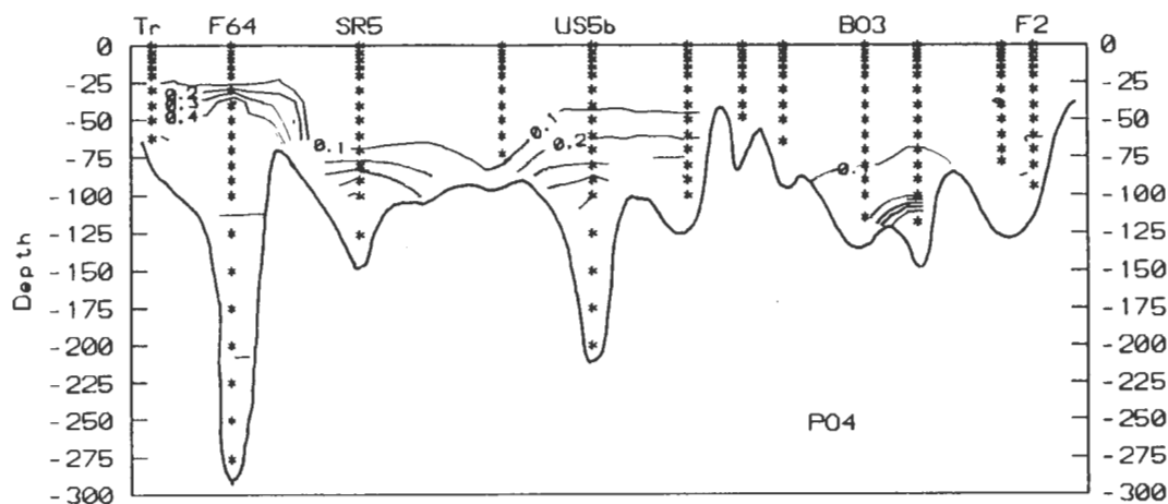
Fig. 39 Fördelningen av \text{PO}_4\text{-P} i snittet genom Bottniska Viken. Avståndet mellan isolinjerna 0.1 \mu\text{mol/l} .
