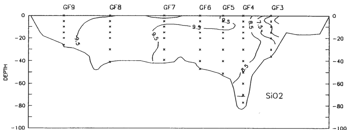
Fig. 5 Fördelningen av silikat i snittet mellan Göteborg och Fredrikshamn. Avståndet mellan isolinjerna är 1 \mu\text{mol/l} .
