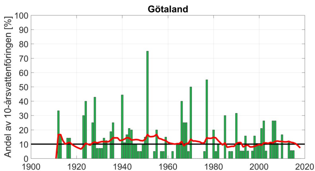
Figur 41 Andelen i % år för år av varje regions vattenförlingsstationer som hade flödestopp med minst 10 års statistisk återkomsttid.
