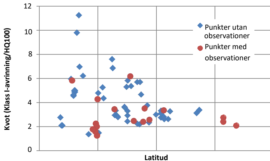
Figur 47 Förhållandet mellan kvoten Klass-I avrinningen/HQ100 samt beräkningspunkten latitud (breddgrad). Nordliga punkter således till höger på x-axeln. Cirkelar avser punkter med mätdata tillgängliga för beräkningen, kvadrater avser punkter utan mätdata
