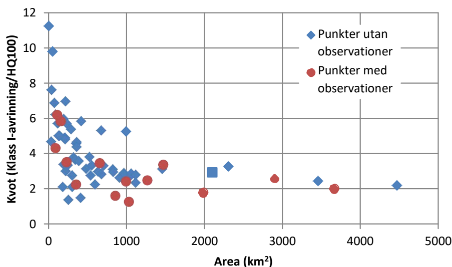
Figur 46 Förhållandet mellan kvoten Klass I-avrinning/100-årsflödet samt avrinningsområdets areal. Cirklar avser punkter med mätdata tillgängliga för beräkningen, kvadrater avser punkter utan mätdata. Överst samtliga punkter, nedre med de största punkterna (från Torne älv) exkluderade.
