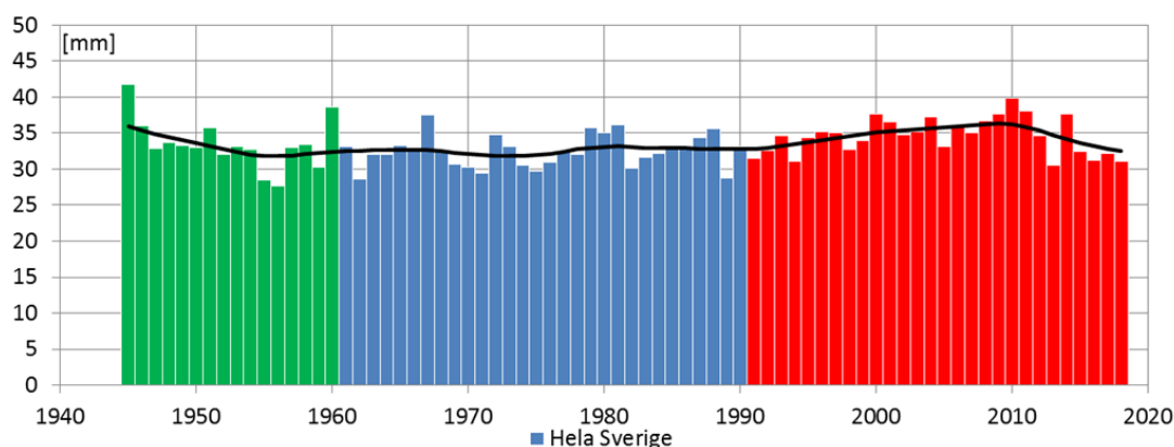
Figur 31 Medelvärdet av årshögsta punktnederbörden över 24 timmar för alla stationer i Sverige för perioden 1945-2018. Den svarta linjen representerar ett flytande 10-årsmedelvärde framtaget med ett Gauss-filter.
