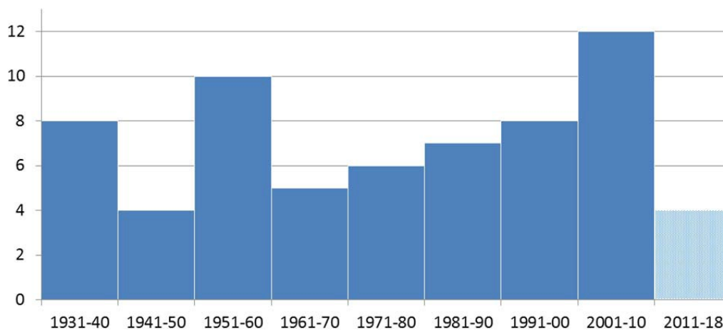
Figur 19 Antalet observerade 24-timmars regn på minst 90 mm i hela Sverige över en yta på 1000 km² per 10-årsperiod.
