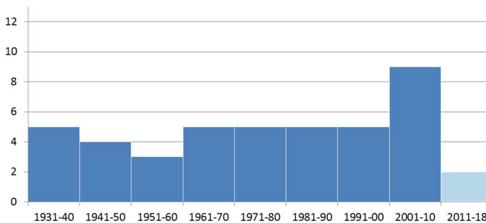
Figur 21 Antalet observerade 24-timmars regn på minst 90 mm i region 4-5 över en yta på 1000 km² per 10-årsperiod.
