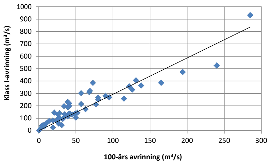
Figur 44 Förhållandet mellan 100-årsflödet och klass-I avrinningen.
