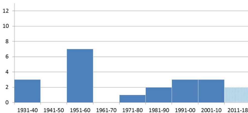
Figur 20 Antalet observerade 24-timmars regn på minst 90 mm i region 1-3 över en yta på 1000 km² per 10-årsperiod.
