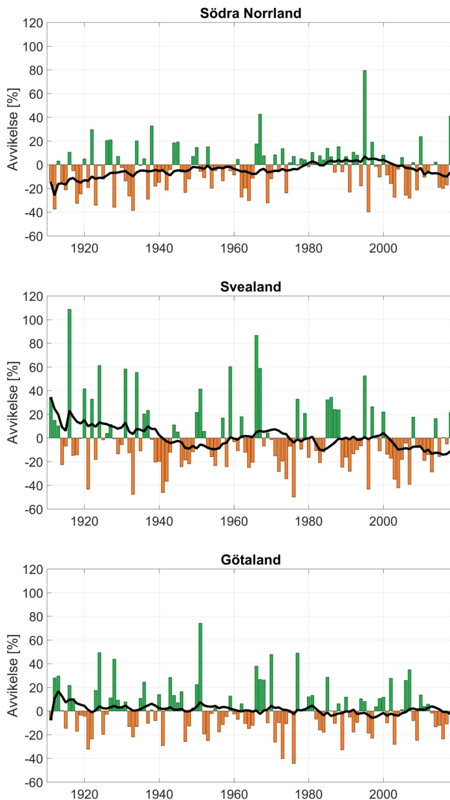
Figur 39 Medelavvikelser från medelvärdet 1961-1990 av årets högsta flödestopp beräknat för vattenföringsstationer uppdelat på 4 regionerna i Figur 7.
