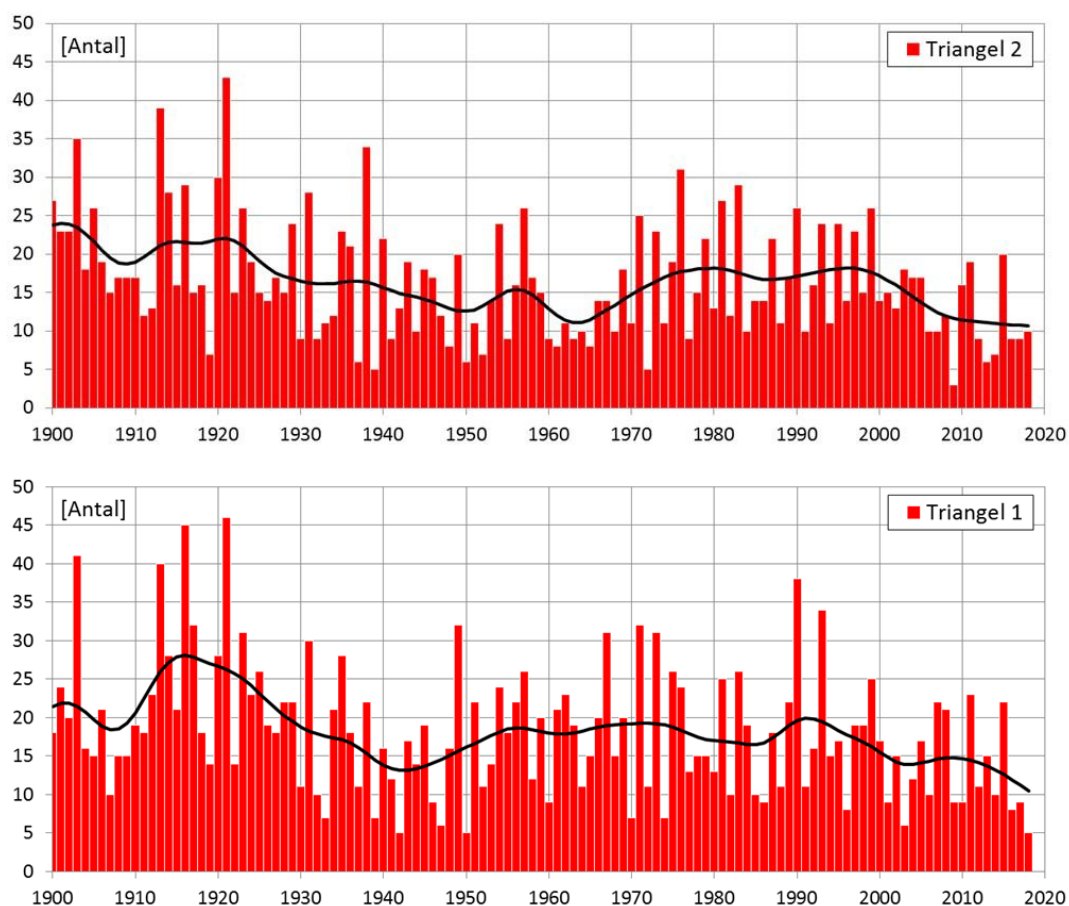
Figur 43 Antal tillfällen i de nio trianglarna i Figur 42 då den geostrofiska vinden varit minst 25 m/s under åren 1940-2018 respektive 1900-2018.
