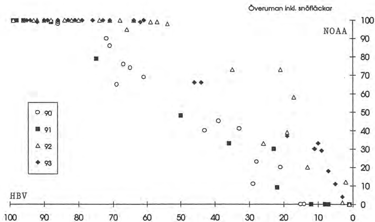
Figur 9a. Överuman 1990, 1991, 1992 och 1993. HBV-modellens snömagasin (procent av maxmagasin) mot snötäckningsgrad (inklusive snöfläckar) enligt NOAA-satellitbilder.
