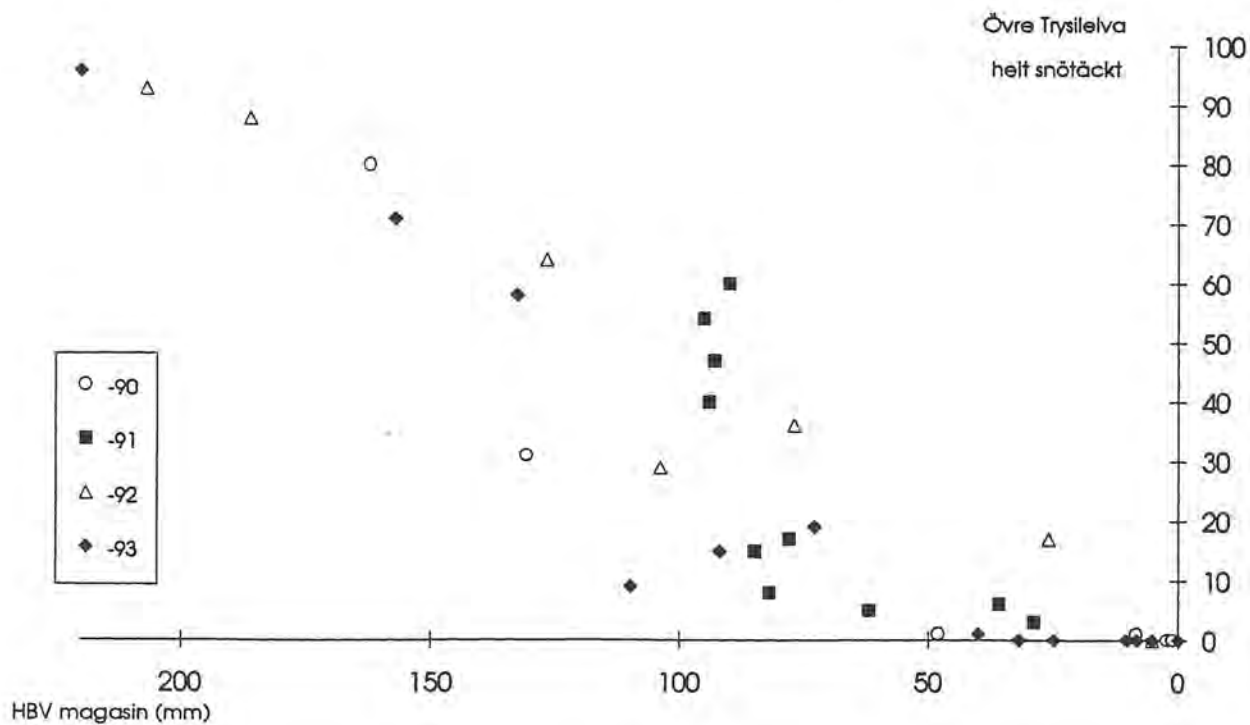
Figur 18b. Övre Trysilälva 1990, 1991, 1992 och 1993. HBV-modellens snömagasin (mm) mot snötäckningsgrad (helt snötäcke) enligt NOAA-satellitbilder.
