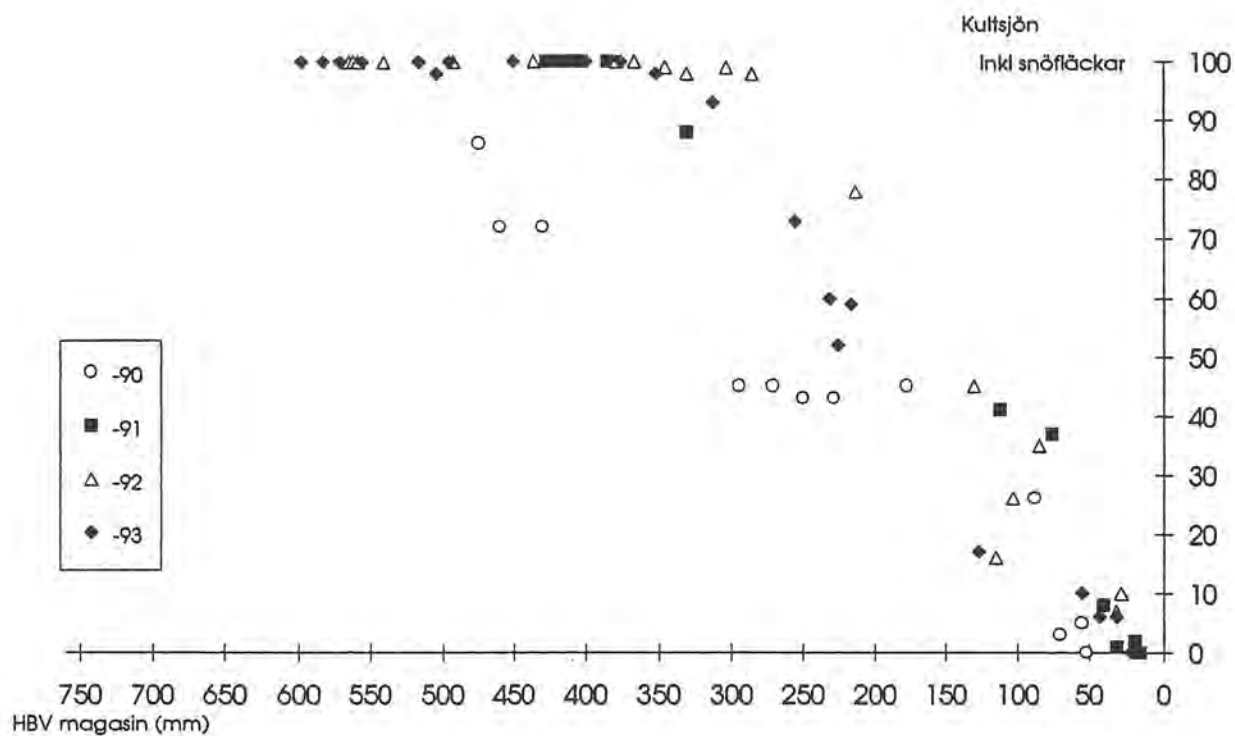
Figur 16a. Kultsjön 1990, 1991, 1992 och 1993. HBV-modellens snömagasin (mm) mot snötäckningsgrad (inklusive snöfläckar) enligt NOAA-satellitbilder.
