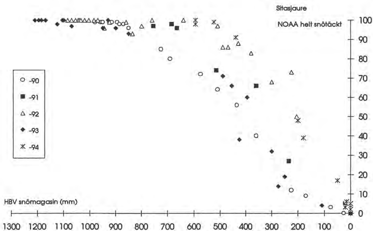
Figur 13b. Sitasjaure 1990, 1991, 1992, 1993 och 1994. HBV-modellens snömagasin (mm) mot snötäckningsgrad (helt snöiäcke) enligt NOAA-satellitbilder.
