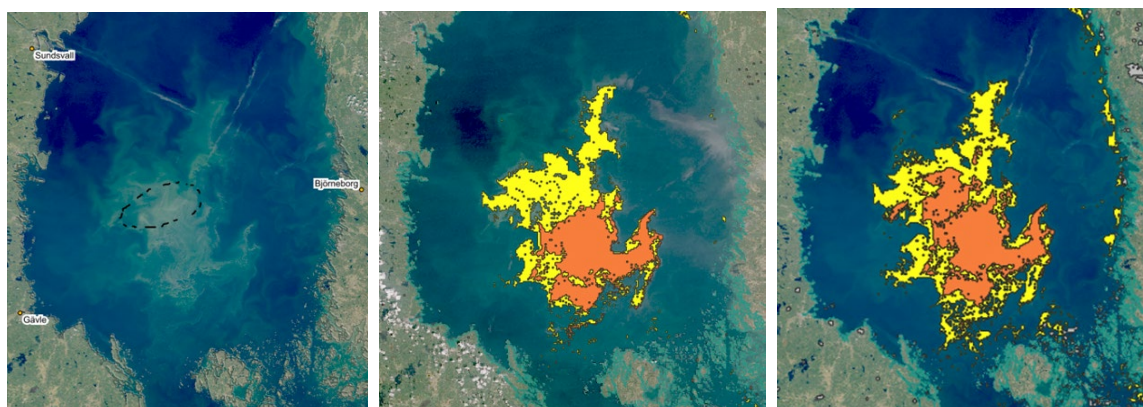
Figur 7. Satellitdata från 2021-07-25.
