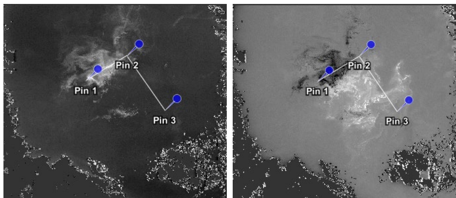
Figur 8. Satellitdata från 2021-07-25.
