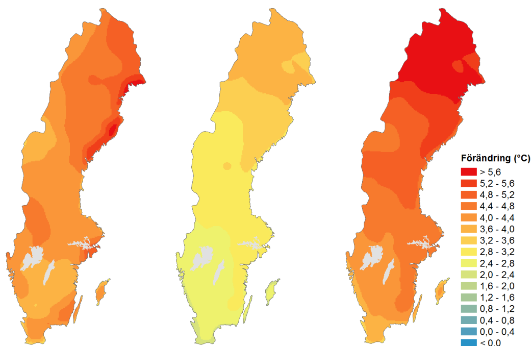
Figur 1. Beräknad förändring av årsmedeltemperatur för perioden 2069-2098 jämfört med perioden 1961-1990, enligt de tidigare beräkningarna med SRES och de nyare med RCP4.5 respektive RCP8.5. Värdena i kartorna är utjämnade för att förenkla tolkningen.
