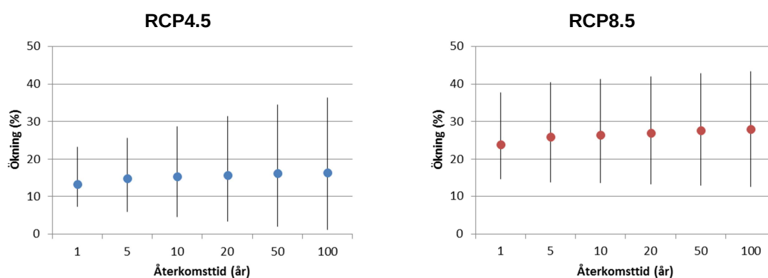
Figur 4. Procentuell förändring av nederbörd med varaktigheten 1 timme mellan perioderna 2069-2098 och 1961-1990 för Västmanlands län. Punkterna representerar medianvärden och vertikala streck visar spridningen mellan de olika modellberäkningarna.
