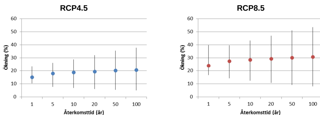
Figur 4. Procentuell förändring av nederbörd med varaktigheten 1 timme mellan perioderna 2069-2098 och 1961-1990 för Stockholms län. Punkterna representerar medianvärden och vertikala streck visar spridningen mellan de olika modellberäkningarna.
