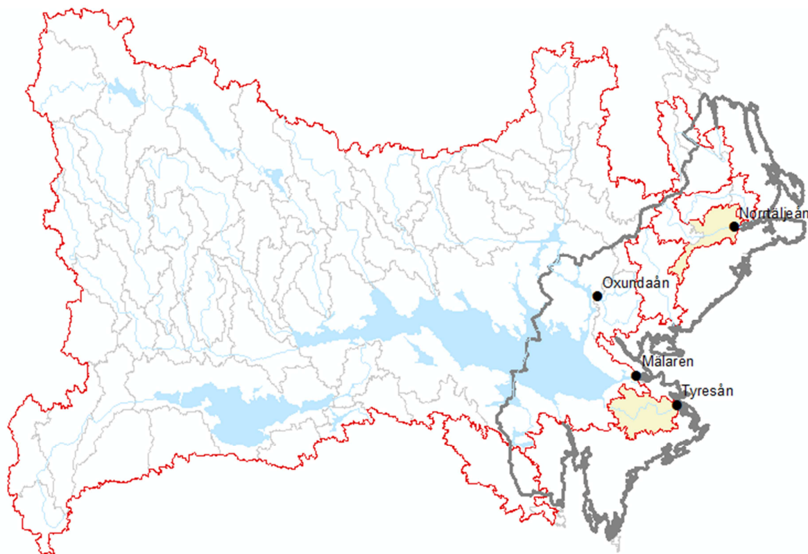
Figur 5. Kartan visar avrinningsområden (röda linjer) och delområden enligt HBV-modellen (ljusgrå linjer). De markerade vattendragspunkterna relaterar till diagrammen över total tillrinning i rapporten. De gulmarkerade områdena avser beräkningarna för lokal tillrinning och markfuktighet. Stockholm län markeras med grå linje.
