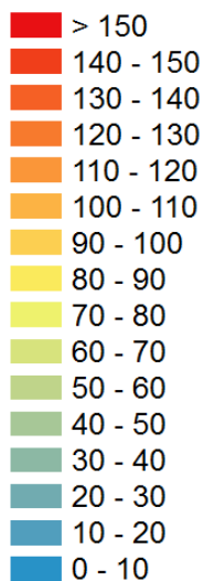
RCP4.5
