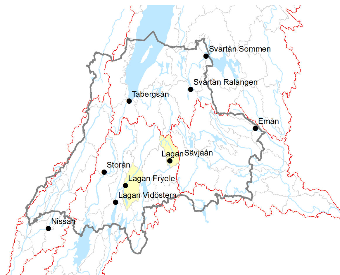
Figur 5. Kartan visar avrinningsområden (röda linjer) och delområden enligt HBV-modellen (ljusgrå linjer). De markerade vattendragspunkterna relaterar till diagrammen över total tillrinning i rapporten. De gulmarkerade områdena avser beräkningarna för lokal tillrinning och markfuktighet. Jönköpings län markeras med mörkgrå linje.
