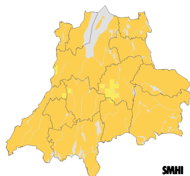
Beräknat 2069-2098
