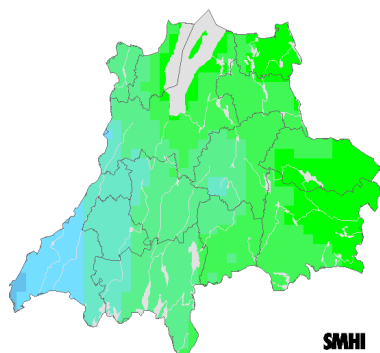
Beräknat 2021-2050
