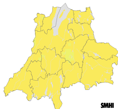
Beräknat 2069-2098
