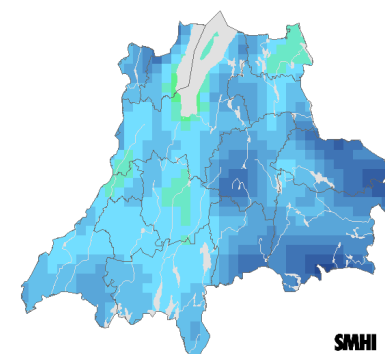
Beräknat 2069-2098
