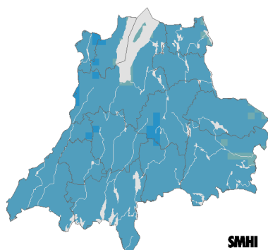
Beräknat 2021-2050
