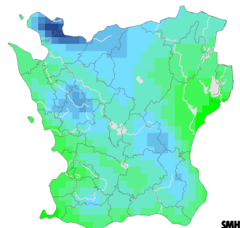
Beräknat 2069-2098
