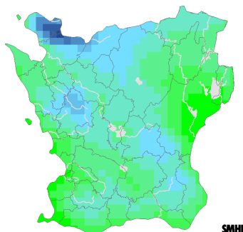
Beräknat 2021-2050
