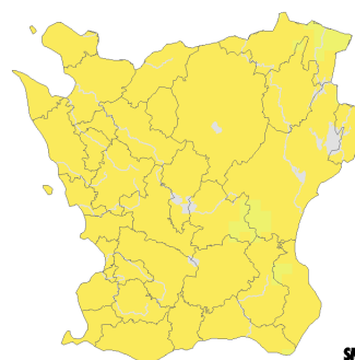
Beräknat 2069-2098
