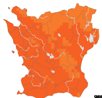
Beräknat 2069-2098
