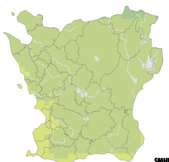
Beräknat 2021-2050
