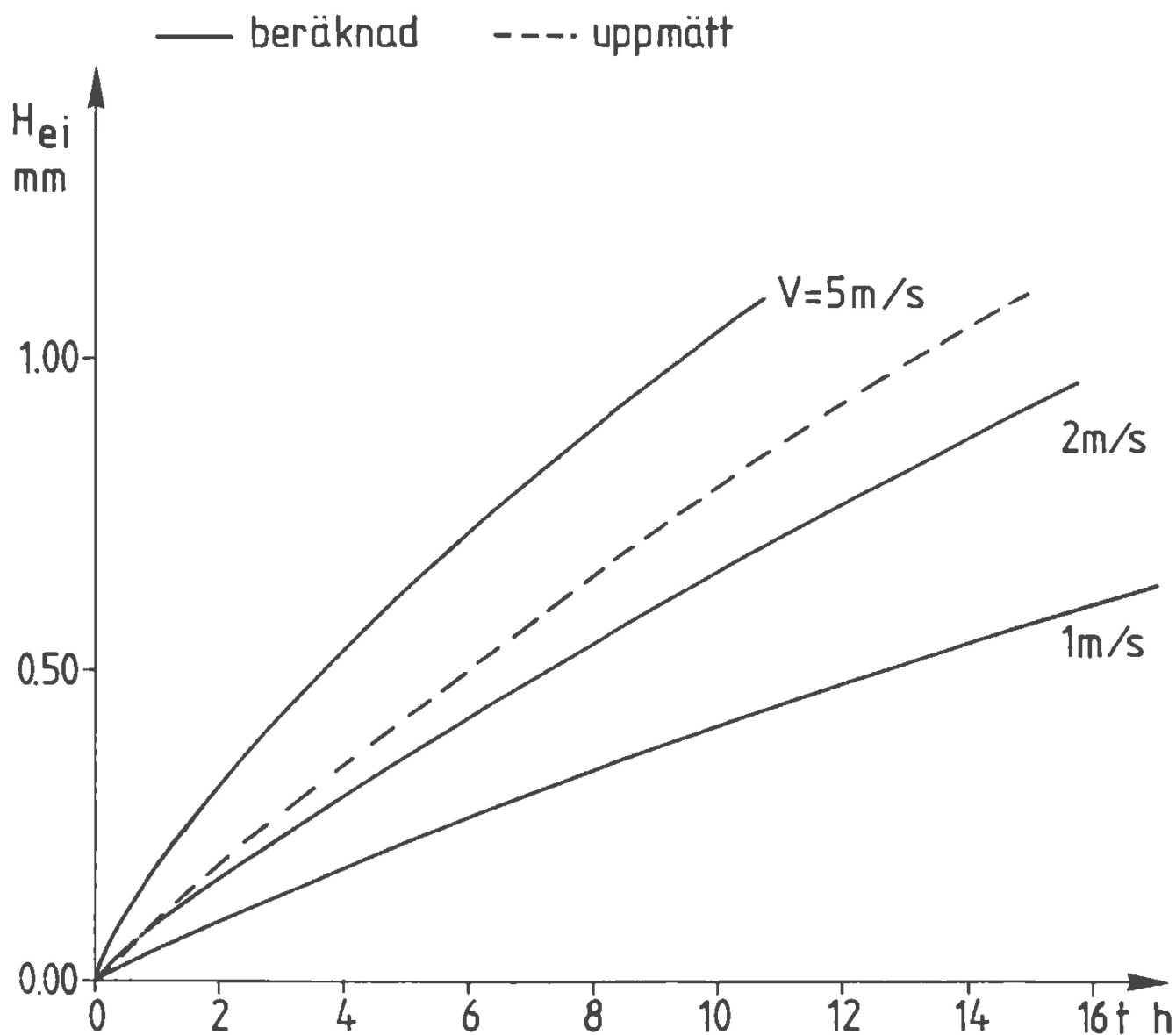
Figur 7. Frysförsluster - avdunstning H_{ei} plottad mot frystiden t vid olika vindhastigheter, lufttemperatur -15^{\circ}\text{C} och relativ fuktighet 100%.
