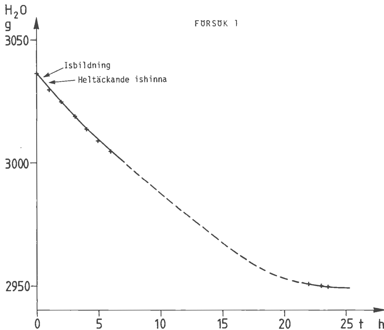
Figur 1. H_2O -vikt i gram plottad mot frystiden t vid lufttemperatur -15^{\circ}C och relativ fuktighet 70 - 80 %.
