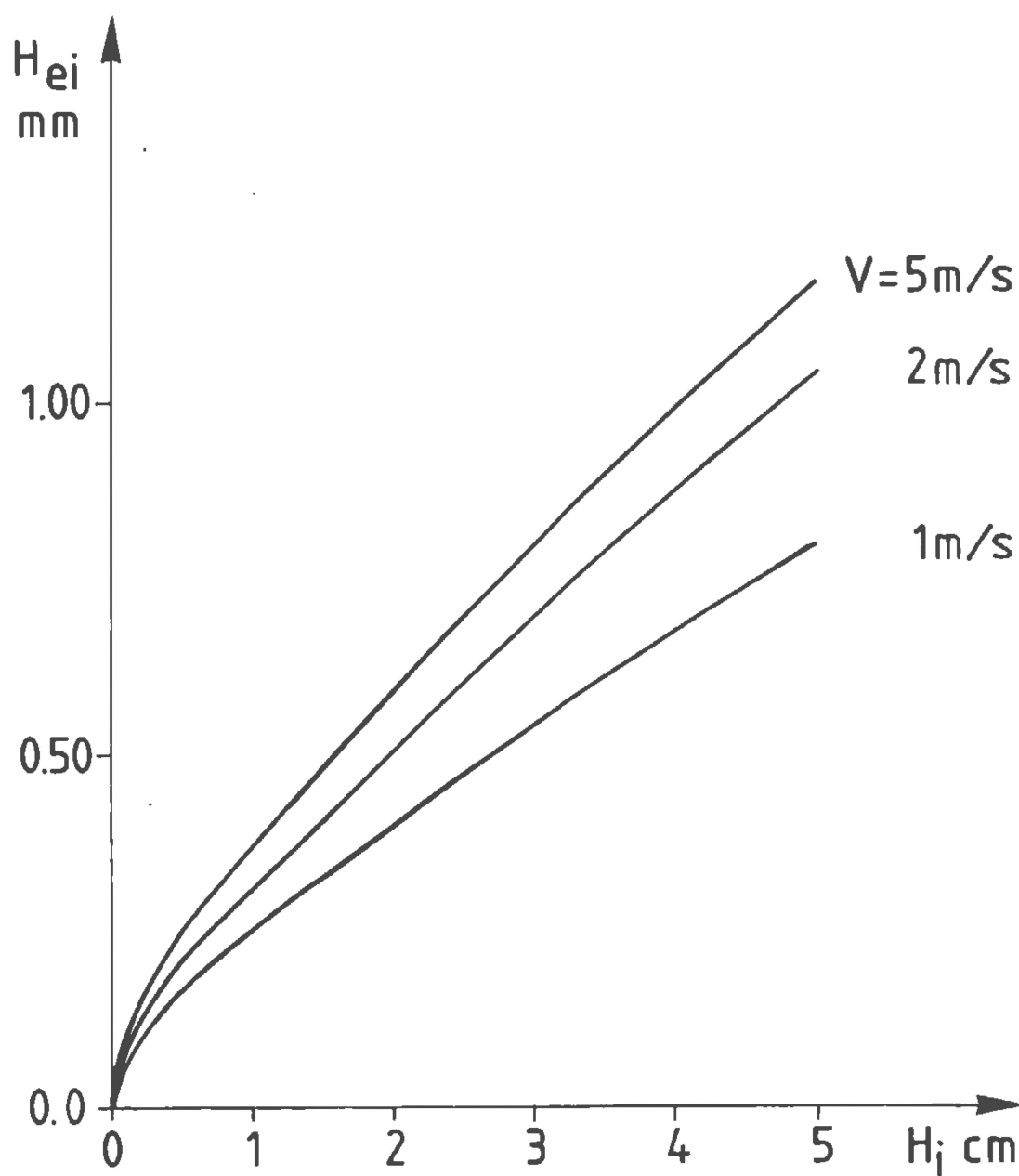
Figur 5. Frys förluster - avdunstning H_{ei} plottad mot istillväxten H_i vid tre olika vindhastigheter, lufttemperatur -150^{\circ}\text{C} och relativ fuktighet 100%.
