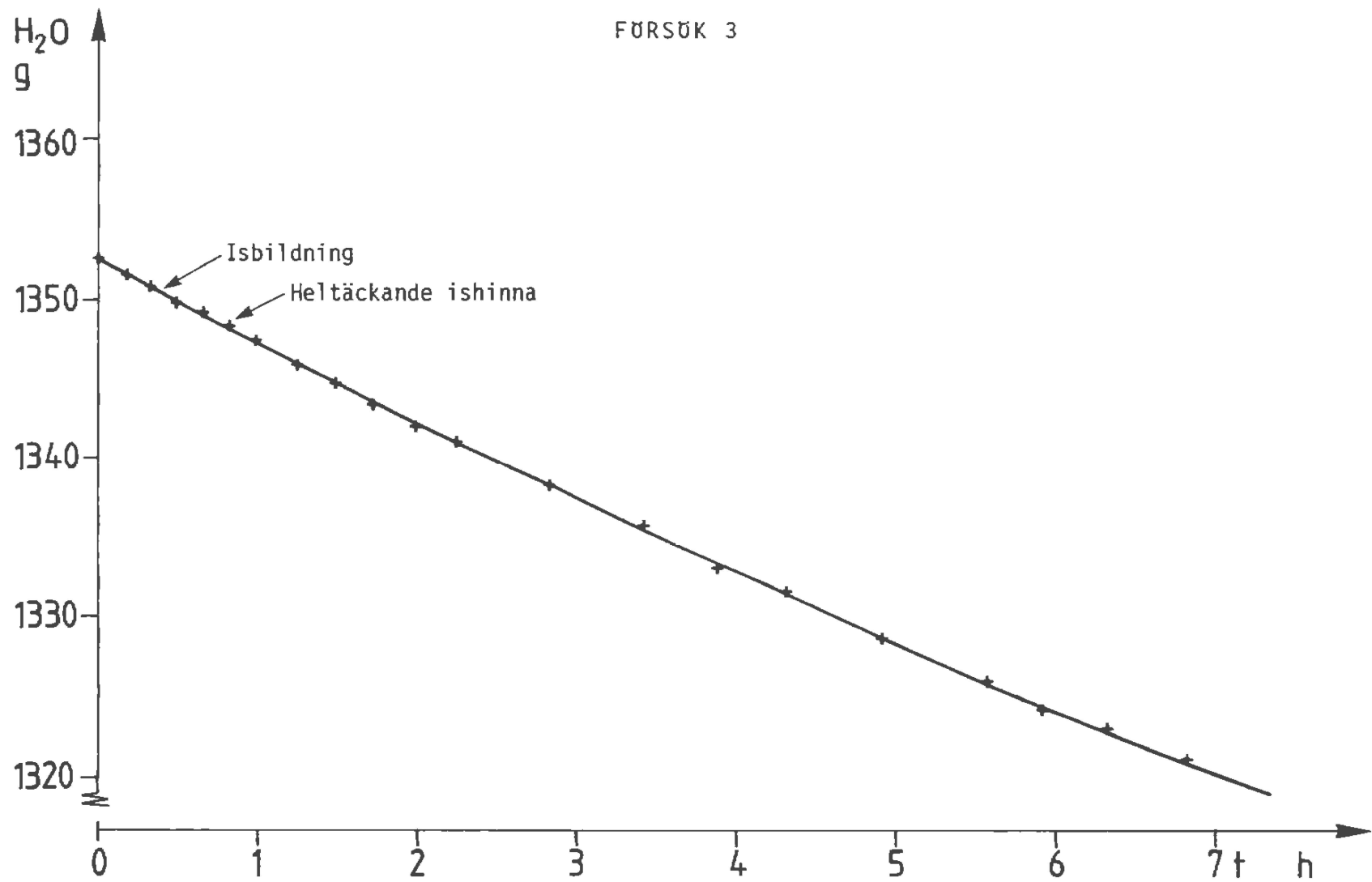
Figur 3. H_2O -vikt i gram plottad mot frystiden t vid lufttemperatur -15^{\circ}C och relativ fuktighet 70 - 80 %
