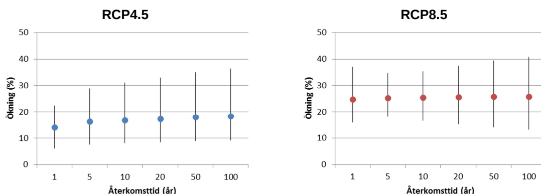
Figur 4. Procentuell förändring av nederbörd med varaktigheten 1 timme mellan perioderna 2069-2098 och 1961-1990 för Blekinge län. Punkterna representerar medianvärden och vertikala streck visar spridningen mellan de olika modellberäkningarna.
