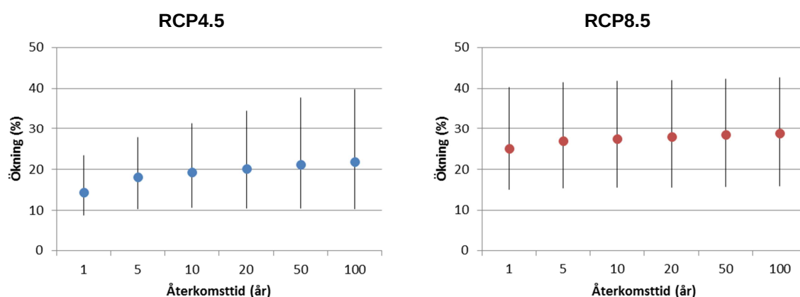
Figur 4. Procentuell förändring av nederbörd med varaktigheten 1 timme mellan perioderna 2069-2098 och 1961-1990 för Gävleborgs län. Punkterna representerar medianvärden och vertikala streck visar spridningen mellan de olika modellberäkningarna.
