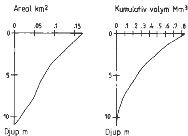
Figur 3: Hypsograf och volymfördelning för sjön Hjorten.
