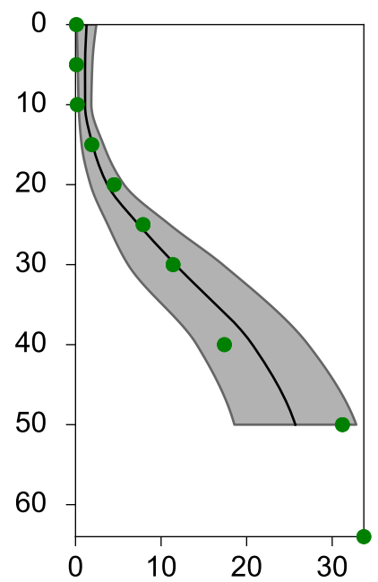
SiO 3 μmol/l
