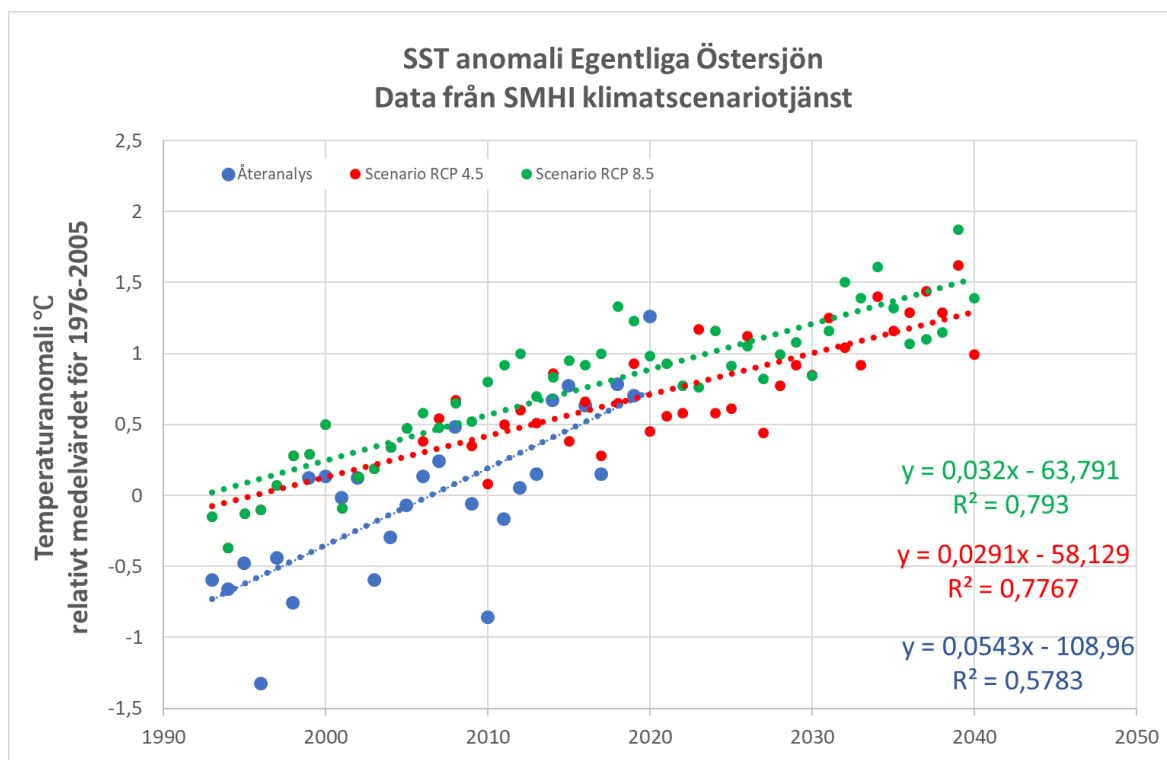
Figur 3. Egentliga Östersjön (inklusive Finska viken och Rigabukten) linjär regression på data från SMHI . Diagrammet visar beräknad förändring av medelvärdet (År) för Ytvattentemperatur (°C) jämfört med referensperioden (medelvärdet för 1976–2005). Trend för återanalys (1993–2020) ca 0,5 °C per årtionde samt för klimatscenario (1993–2040) RCP4,5 ca 0,3 °C per årtionde och RCP8,5 ca 0,3 °C per årtionde.
