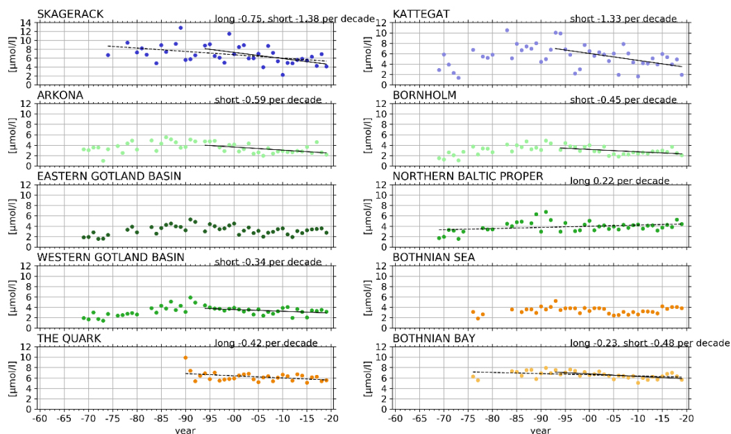
Figur 16. Figurer från Wesslander et al. (2020) . SMHI uppskattade trender för totalkväve (överst) och löst oorganiskt kväve (nederst) i ytvattnet (0–10m) under vintern. En linje visas när p-värdet för lutningen är \leq 0,05 . Streckad linje visas för de längre tidsserierna och heldragen linje för tidsserien efter 1994.
