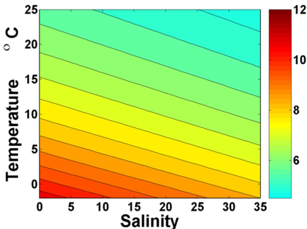
Figur 15. Syremättad (färgskala i ml/l) vid olika temperatur och salthalt. Baserad på formuleringar som används för RCO–SCOBI modellen (se referenser i Eilola et al 2009 ).
