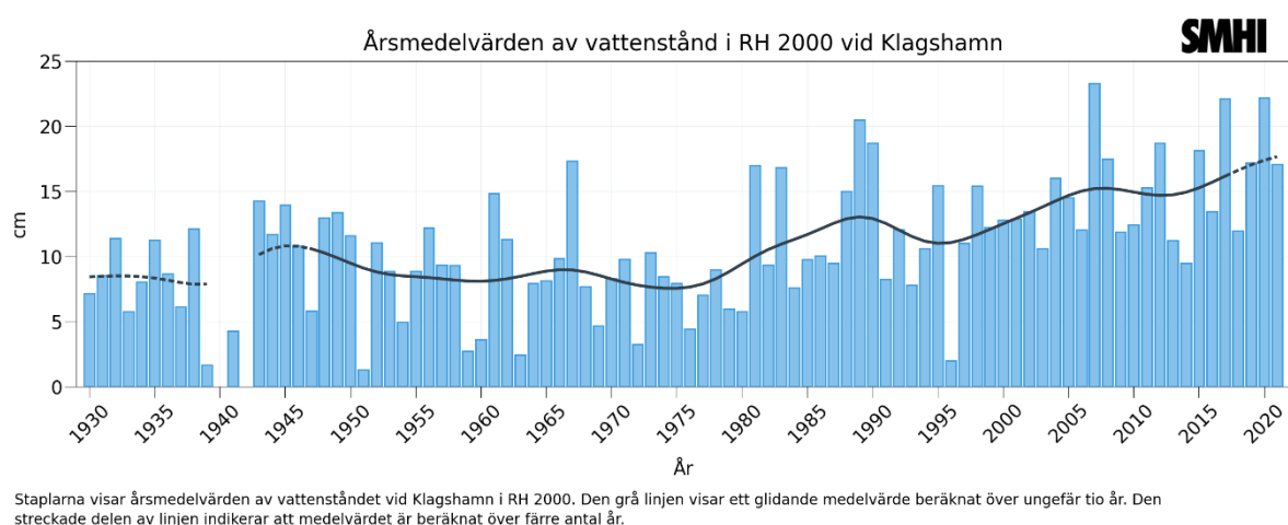
Figur 10. Exempel på vattenstånds förändringar vid Ratan i Bottenviken och Klagshamn i Skåne med landhöjning inkluderad. Diagram nedladdat från klimatindikator för havsnivå .
