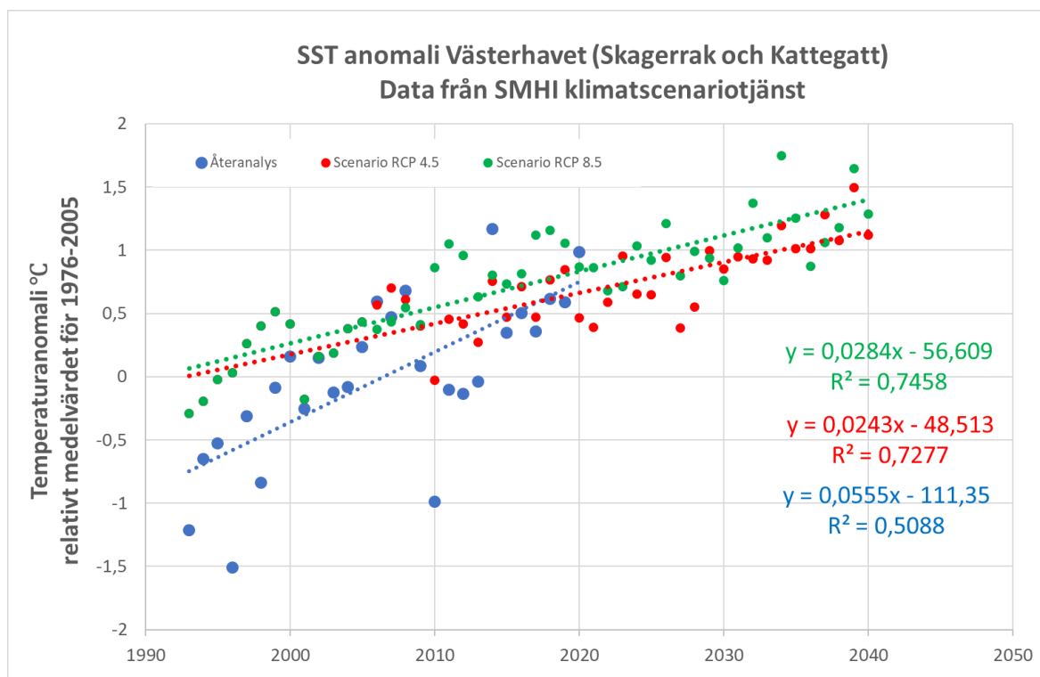
Figur 4. Västerhavet linjär regression på data från SMHI . Diagrammet visar beräknad förändring av medelvärdet (År) för Ytvattentemperatur (°C) viken jämfört med referensperioden (medelvärdet för 1976–2005). Trend för återanalys (1993–2020) ca 0,6 °C per årtionde samt för klimatscenario (1993–2040) RCP4,5 ca 0,2 °C per årtionde och RCP8,5 ca 0,3 °C per årtionde.
