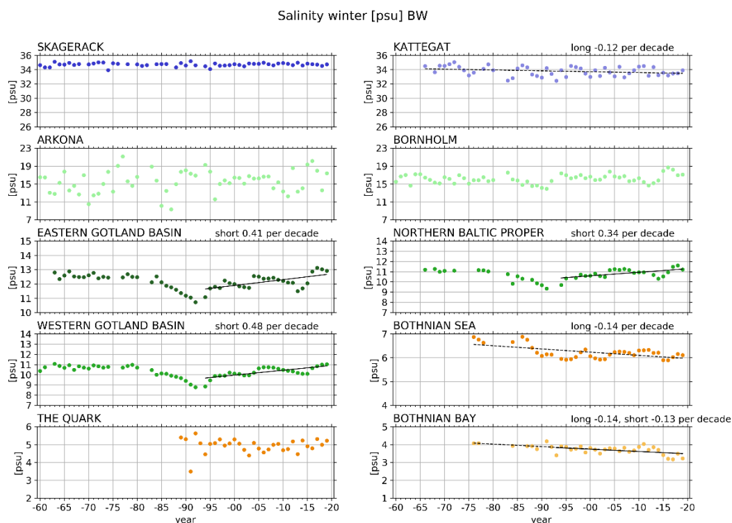
Figur 5. Figurer från Wesslander et al. (2020) . SMHIs trendanalyser baserat på data från 1960- och 1970-talet. Ytvattensalthalt sommar (över) och vinter (mitten). Salthalt vinter vid botten (nederst). Skagerrackdata visar ingen trend medan Kattegatts sommarvärden visar en negativ trend. En linje visas när p -värdet för lutningen är \leq 0,05 . Streckad linje visas för de längre tidsserierna och heldragen linje för tidsserien efter 1994.
