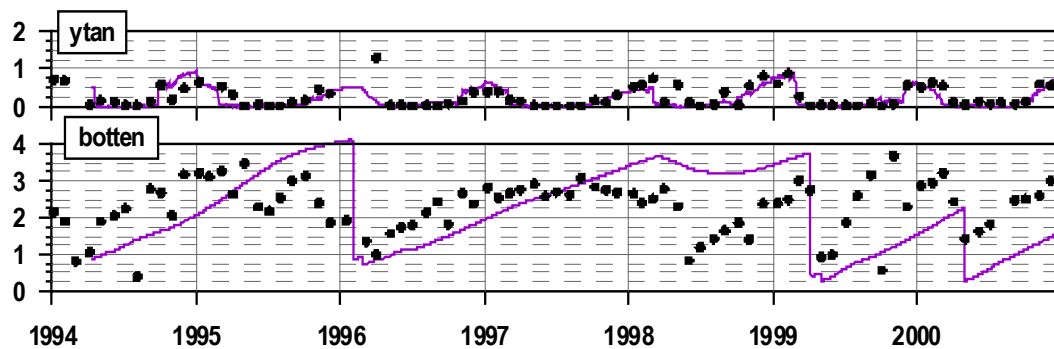
Figur 20. Jämförelse mellan modellerad fosfathalt ( \mu\text{mol/l} ) från B27 och mätdata från stationerna Björkholmen på 5m djup respektive Alsbäck på 110m djup. Lila linje visar modellresultat och svarta punkter observationer.
