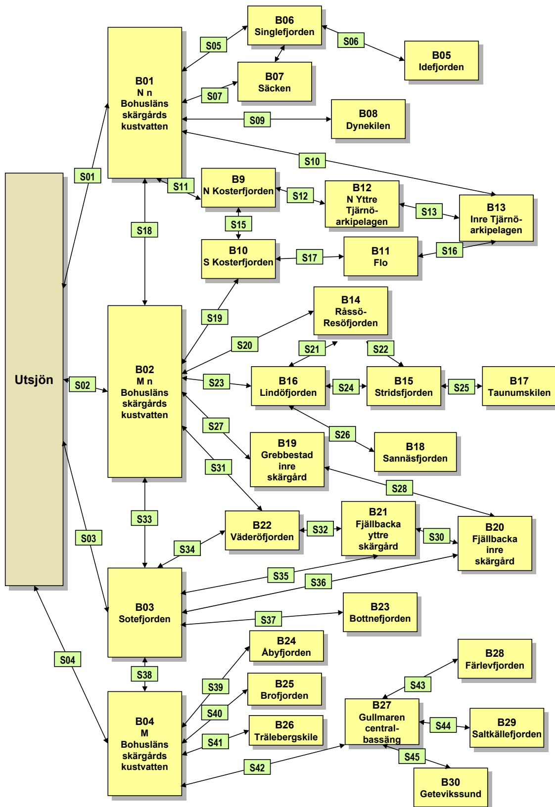
Figur 6. Schematisk beskrivning över bassängindelningen samt kopplingar mellan delbassängerna i modelluppsättningen för den norra delen av Bohusläns skärgård.
