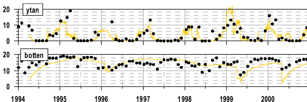
Figur 19. Jämförelse mellan modellerad nitrathalt (µmol/l) från B27 och mätdata från stationerna Björkholmen på 5m djup respektive Alsbäck på 110m djup. Gul linje visar modellresultat och svarta punkter observationer.
