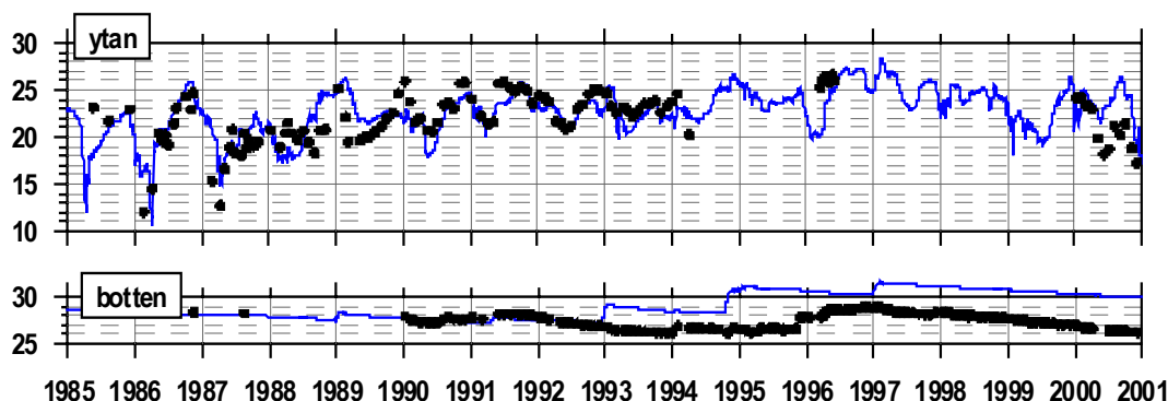
Figur 53. Jämförelse mellan modellerad salthalt (PSU) från B07 och mätdata från station Koljöfjorden . Blå linje visar modellresultat och svarta punkter observationer på 0 respektive 40 m djup.
