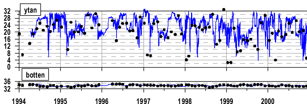
Figur 21. Jämförelse mellan modellerad salthalt (PSU) från B29 och mätdata från stationen Björkholmen på 0 resp. 50m. Blå linje visar modellresultat och svarta punkter observationer.
