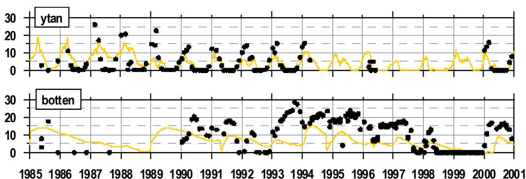
Figur 56. Jämförelse mellan modellerad nitrathalt ( \mu\text{mol/l} ) från B07 och mätdata från station Koljöfjorden . Gul linje visar modellresultat och svarta punkter observationer på 0 respektive 40 m djup.
