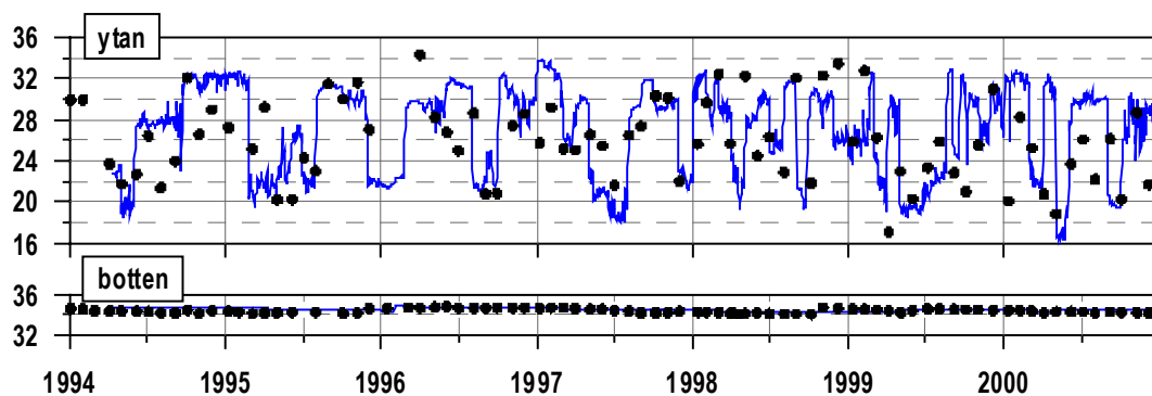
Figur 16. Jämförelse mellan modellerad salthalt (PSU) från B27 och mätdata från stationerna Björkholmen på 5m djup respektive Alsback på 110m djup. Blå linje visar modellresultat och svarta punkter observationer.
