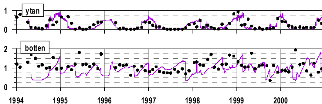
Figur 25. Jämförelse mellan modellerad fosfathalt ( \mu\text{mol/l} ) från B29 och mätdata från stationen Björkholmen på 0 resp. 50m. Lila linje visar modellresultat och svarta punkter observationer.
