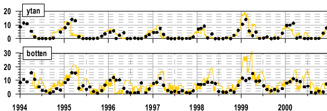
Figur 29. Jämförelse mellan modellerad nitrathalt ( \mu\text{mol/l} ) från B25 och mätdata från stationen Stretudden . Gul linje visar modellresultat på 0 respektive på 31 m djup (modellens maximala djup i denna bassäng) och svarta punkter observationer i ytan och mellan 30 och 40 m djup.
