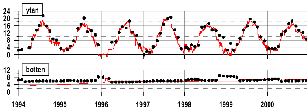
Figur 17. Jämförelse mellan modellerad temperatur (°C) från B27 och mätdata från stationerna Björkholmen på 5m djup respektive Alsback på 110m djup. Röd linje visar modellresultat och svarta punkter observationer.
