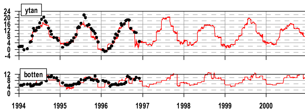
Figur 12. Jämförelse mellan modellerad temperatur (°C) från B04 och mätdata från station Tröskeln . Röd linje visar modellresultat och svarta punkter observationer på 0 respektive 50 m.
