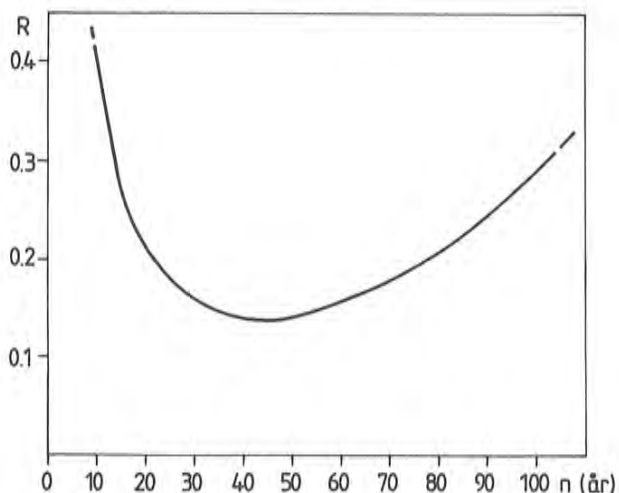
Riskfunktionens (definierad i texten) variation med längden av den period för vilken man beräknar ett medelvärde.
