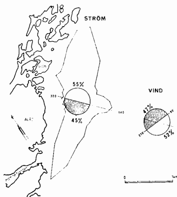
Fördelning av vind- och strömriktningar vid Simevarp under perioden 75-09-24--76-10-27
