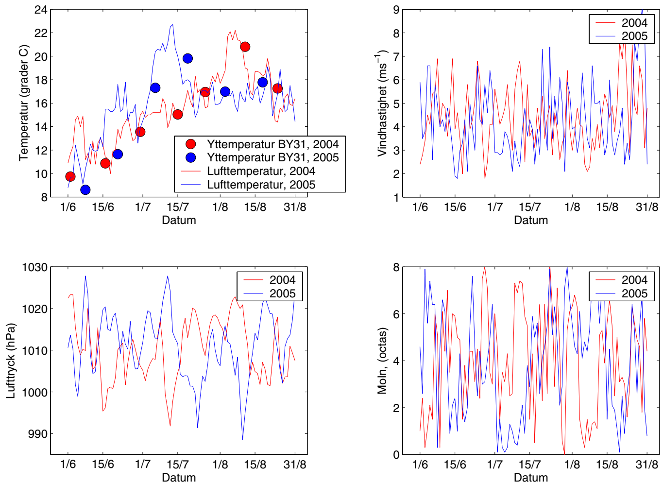
Figur 9. Jämförelse mellan åren 2004 och 2005. Överst till vänster: Dygnsmedel för lufttemperatur vid Gotska Sandön och ytvattentemperatur vid BY31 (se karta figur 7). Överst till höger: Dygnsmedel för vindhastighet. Underst till vänster: Dygnsmedel för lufttryck. Underst till höger: Dygnsmedel för molnmängd, presenteras i åttondelar täckta av himlen täckta av moln (octas).
