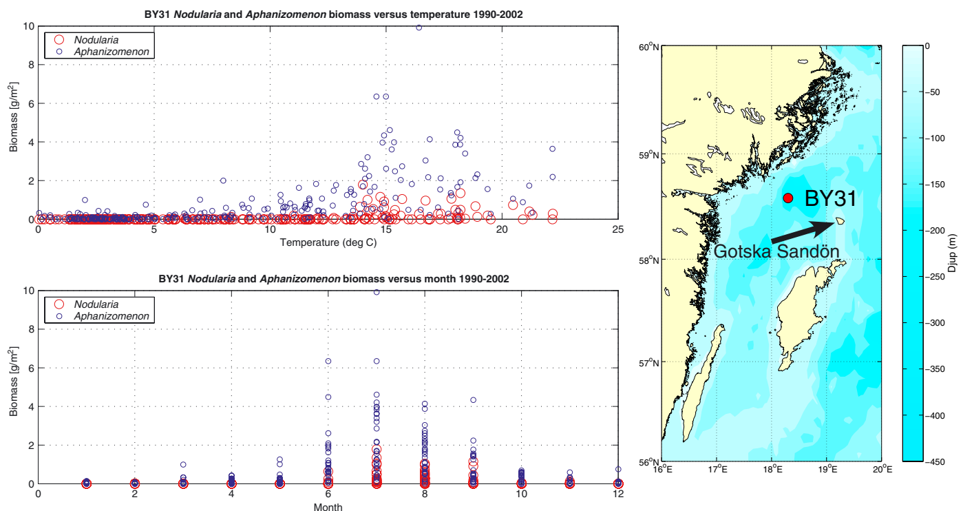
Figur 7. Till vänster: Biomassa av Nodularia och Aphanizomenon mot ytttemperatur och månad vid Landsortsdjupet (station BY31). Data från nationell miljöövervakning utförd av Stockholms Marina Forskningscentrum. Till höger: Karta som visar station BY31 samt Gotska Sandön.
