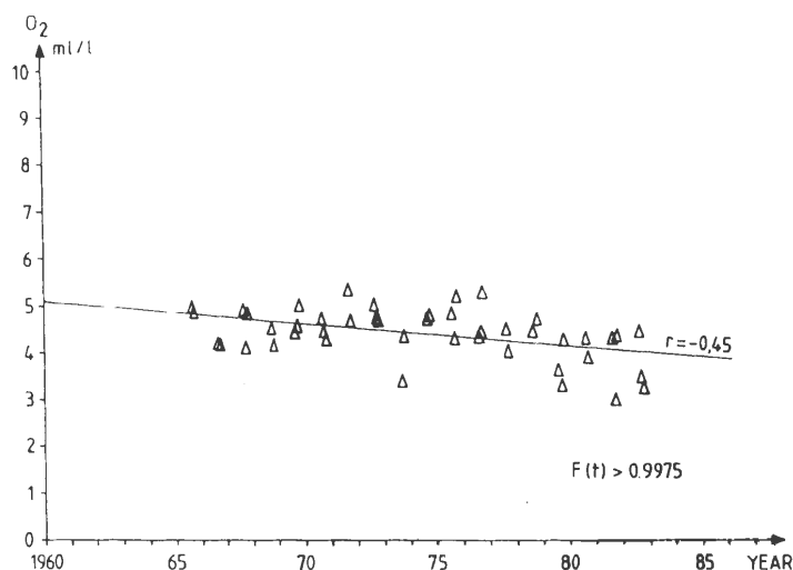
Fig.15. Månadsmedelvärden för syrgas i Kattegatts djupvatten för perioden augusti-oktober 1965-1982. Trenden är baserad på lineär regression (Rydberg 1987).
