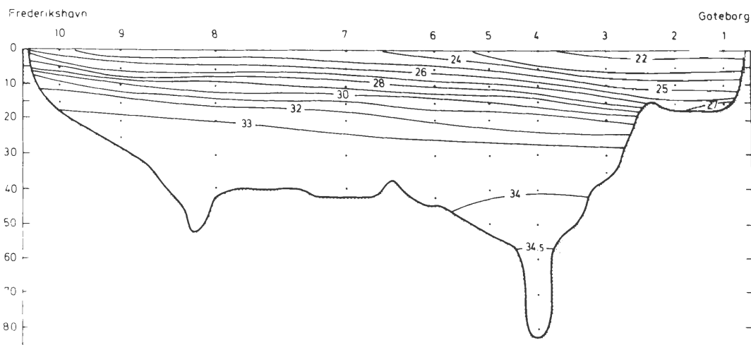
Fig. 8. Medelsalthaltfördelning 1975 -1977. Tvärsnitt genom Kattegatt. Fredrikshamn - Göteborg. (Från Thorstensson 1980).
