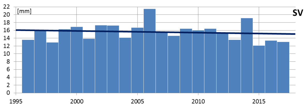
Figur 2. Medelvärdet av årets högsta 1-tim regnvolym av varje regions samtliga stationer. Regioner (uppifrån och ner): N, M, Sö, SV.
