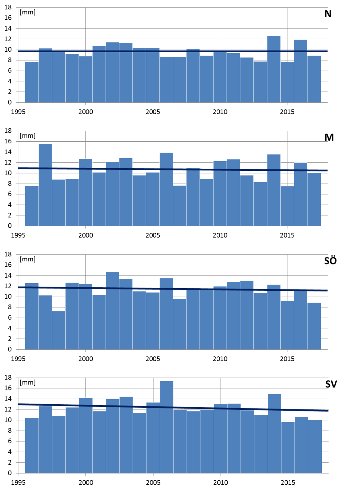
Figur 1. Medelvärde av årets högsta 30-min regnvolym av varje regions samtliga stationer. Regioner (uppifrån och ner): N, M, SÖ, SV.
