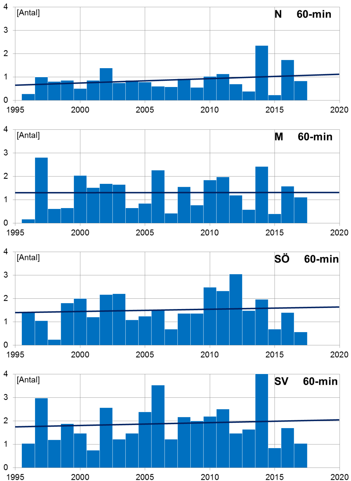
Figur 6. Medelvärde av frekvensen regnvolymer > 13.8 mm/1 tim i varje regions samtliga stationer. Regioner (uppifrån och ner): N, M, SÖ, SV.
