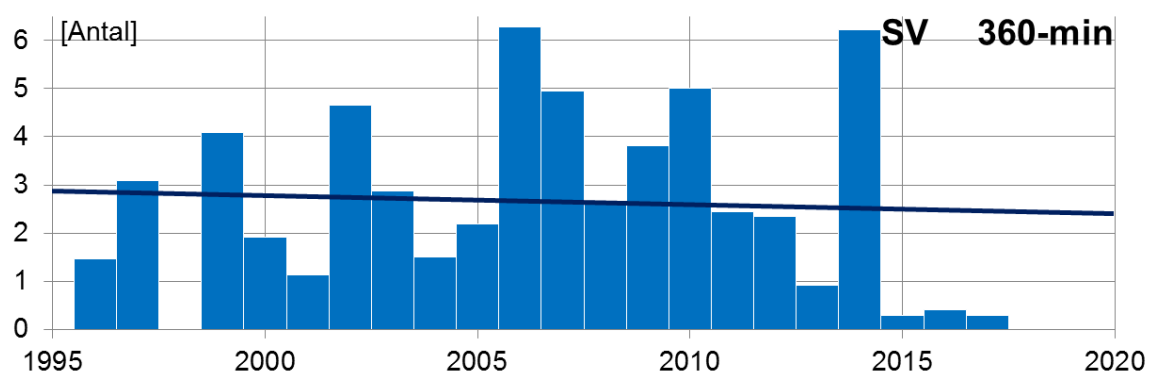
Figur 8. Medelvärde av frekvensen regnvolymer > 33.6 mm/6 tim i varje regions samtliga stationer. Regioner (uppfån och ner): N, M, SÖ, SV.
