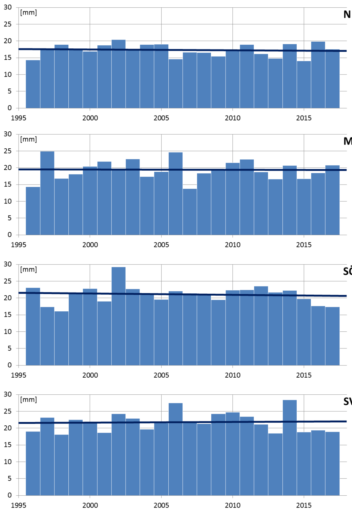
Figur 3. Medelvärdet av årets högsta 3-tim regnvolym av varje regions samtliga stationer. Regioner (uppiifrån och ner): N, M, SÖ, SV.
