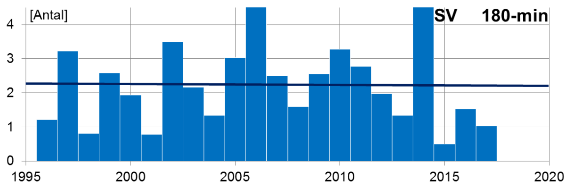
Figur 7. Medelvärde av frekvensen regnvolym > 24.6 \text{ mm}/3 \text{ tim} i varje regions samtliga stationer. Regioner (uppifrån och ner): N, M, SÖ, SV.
