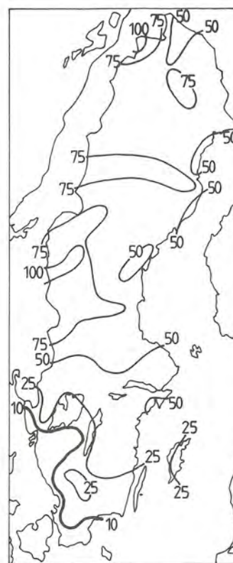
Fig. 6.1c Snödjup. (82-02-19 06Z)
