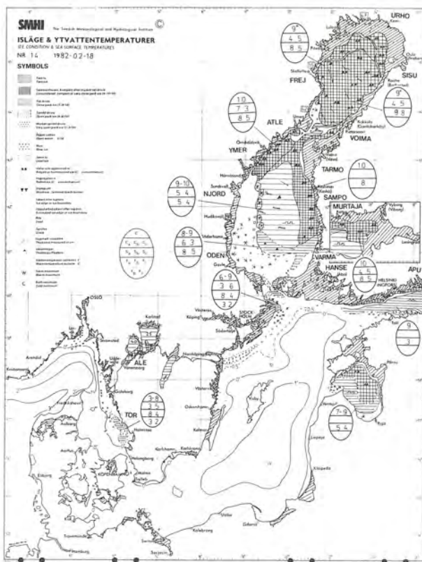
Fig. 6.1b Iskarta. (82-02-18)
