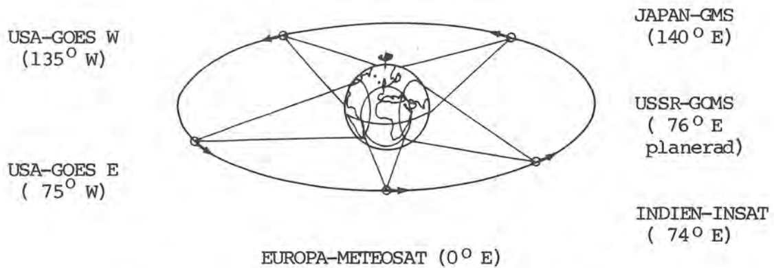
Fig. 2.2 Det GEOSTATIONÄRA satellit-systemet.
