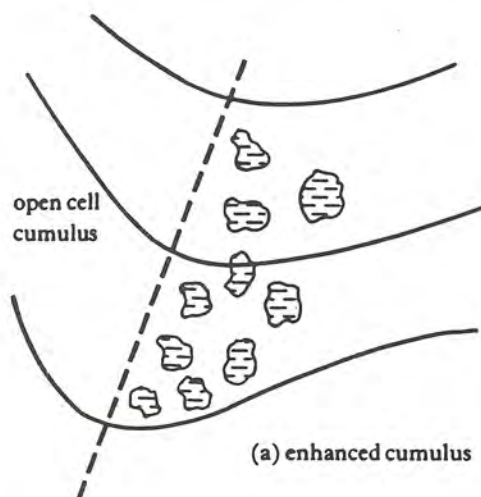
Fig. 5.34 Förstärkt Cumulus-aktivitet.
