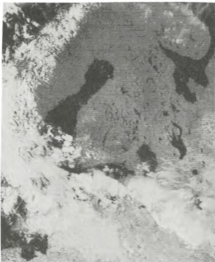
a. VIS
