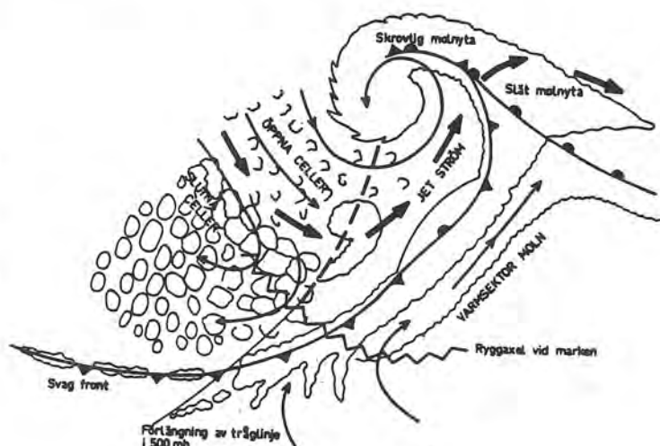
Fig. 5.1b Schematisk bild av en ockluderad frontstörning.
