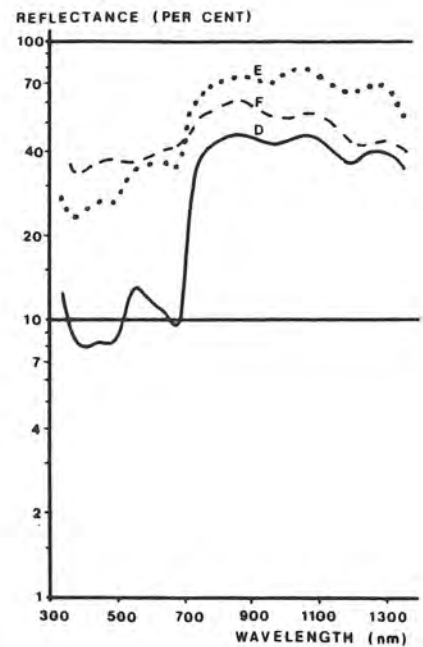
Fig. 2.20 Spektrala reflekti- viteten hos:
