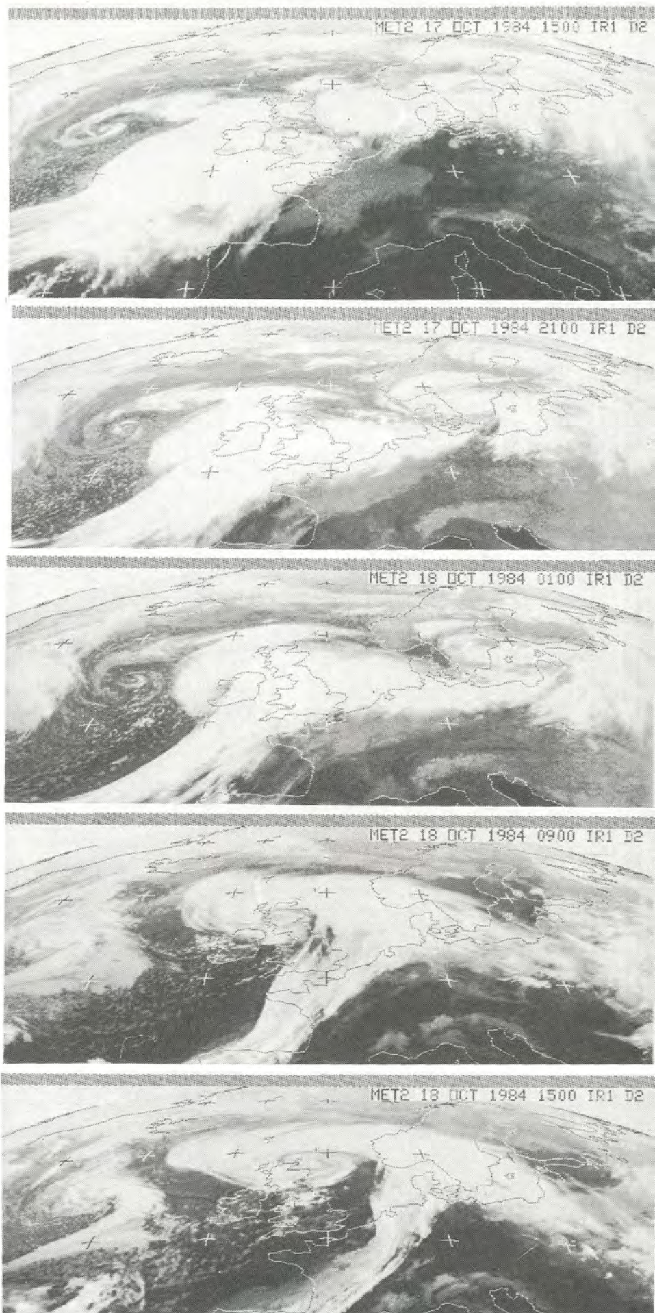
Fig. 5.25a Meteosat IR.
