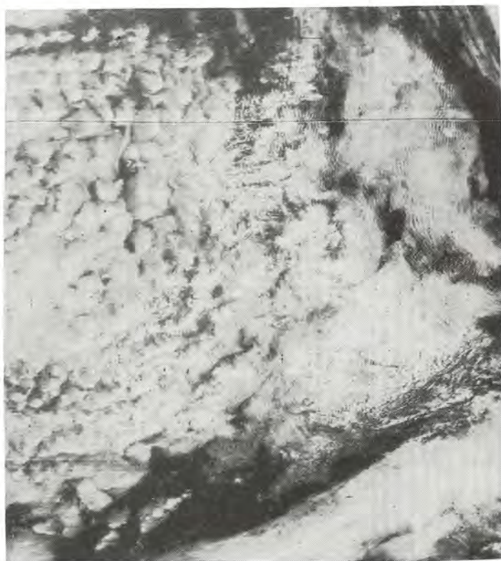
Fig. 3.11 STRATOCUMULUS.
