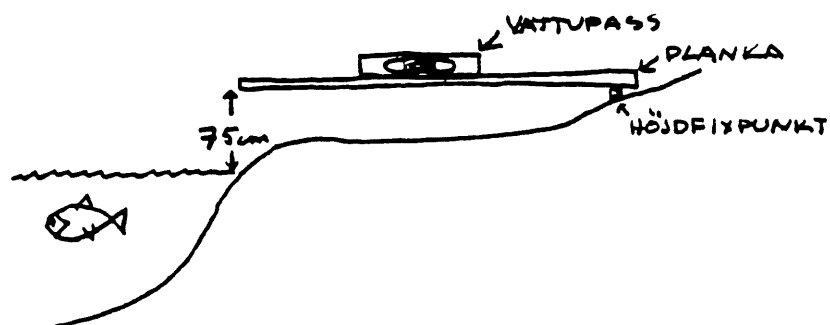
Fig. 2. Höjdbestämning med planka.
