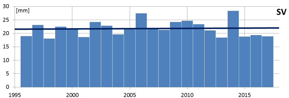
Figur 3. Medelvärdet av årets högsta 3-tim regnvolym av varje regions samtliga stationer. Regioner (uppifrån och ner): N, M, SÖ, SV.
