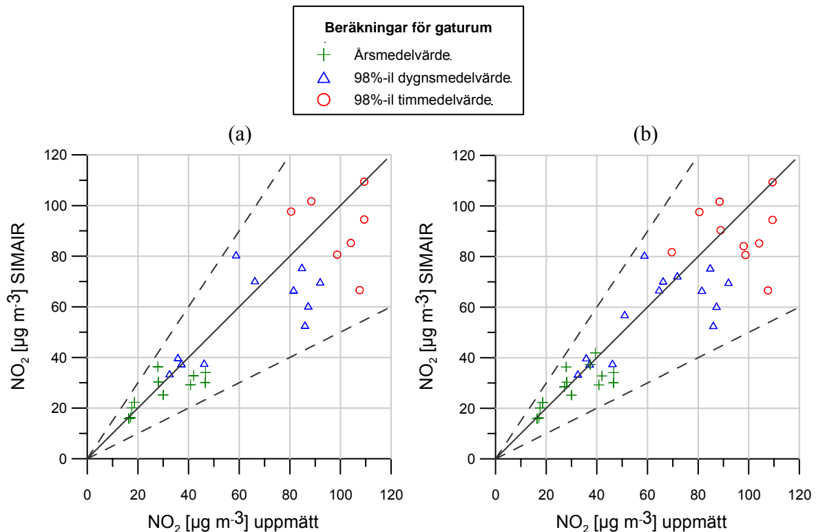
Figur 6. Jämförelse mellan uppmätta och beräknade halter av \text{NO}_2 ( \mu\text{g m}^{-3} ) uttryckta som statistiska haltmått enligt miljökvalitetsnormerna. Helledragen linje anger förhållandet 1:1 och streckade linjer \pm 50\% . Numeriska värden återfinns i Tabell 11. (a) Jämförelse enbart för gaturum i denna studie. (b) Jämförelse för gaturum i denna studie samt tidigare valideringar av SIMAIR (Omstedt och Gidhagen, 2007; Omstedt, 2008).
