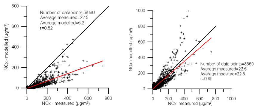
Figur 4. Jämförelse mellan uppmätta och beräknade timmedelhalter av \text{NO}_x ( \mu\text{g m}^{-3} ) för Stadsbibliotekets tak i Umeå år 2003. Till vänster visas beräkningsresultat (urban bakgrund) från SIMAIR utan klimatkorrigering och till höger visas motsvarande figurer med statistisk korrektion genom regressionsanalys, från Omstedt och Gidhagen (2007).
