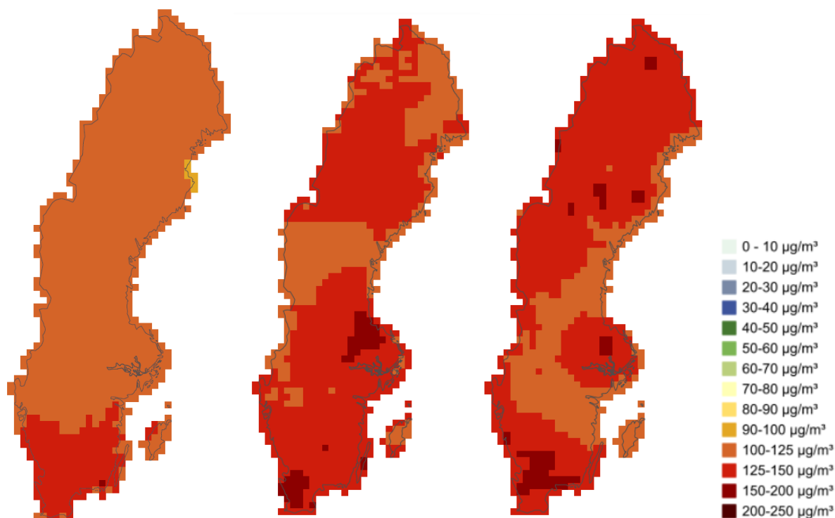
Figur 27. Årets maximala åttatimmarsmedelvärde år 2017 (vänster), 2018 (mitten) och 2019 (höger) för halt i luft av marknära ozon.
