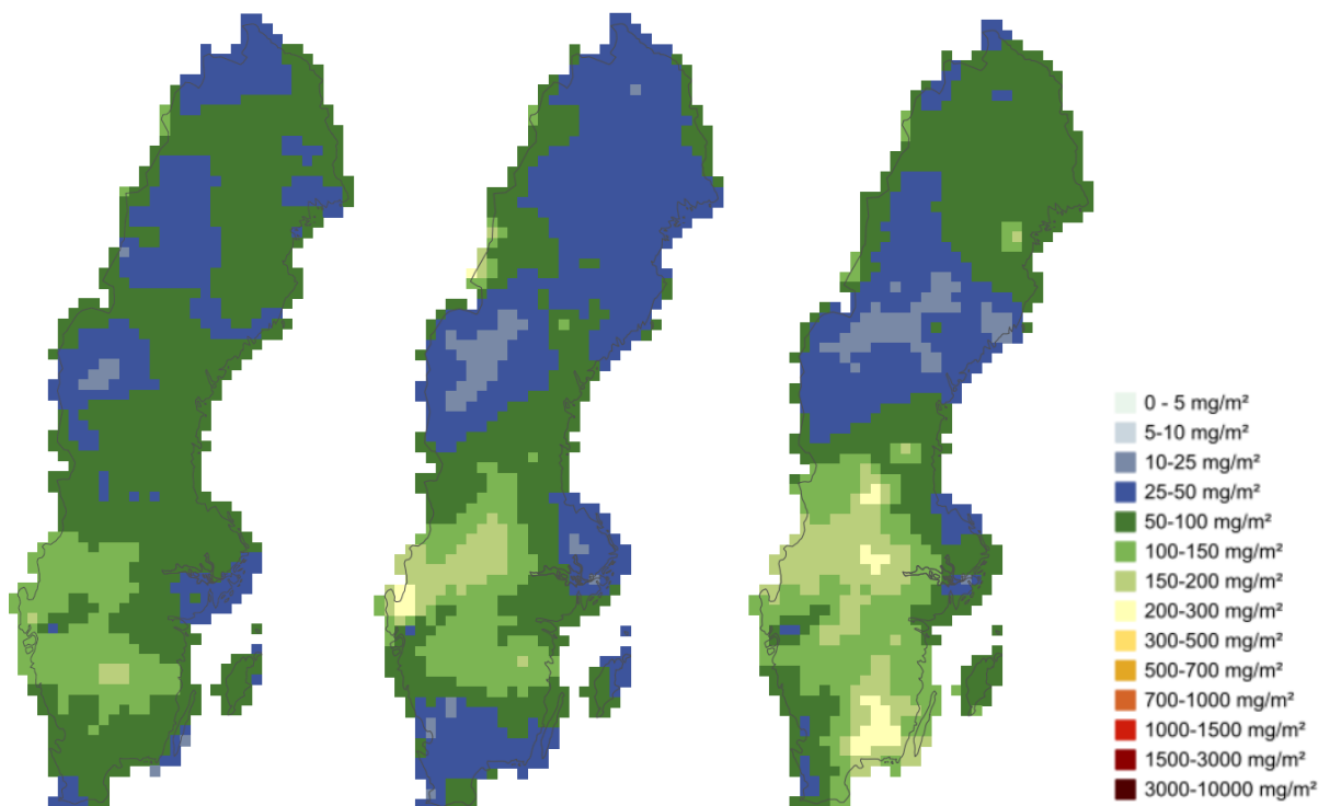
Figur 23. Våtdeposition av kalium år 2017 (vänster), 2018 (mitten) och 2019 (höger). Enhet: mg K m -2 .
