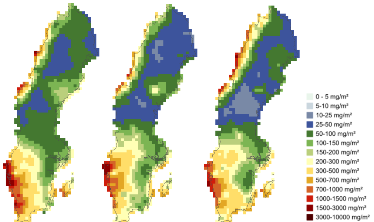
Figur 25. Våtdeposition av natrium år 2017 (vänster), 2018 (mitten) och 2019 (höger). Enhet: mg Na m -2 .
