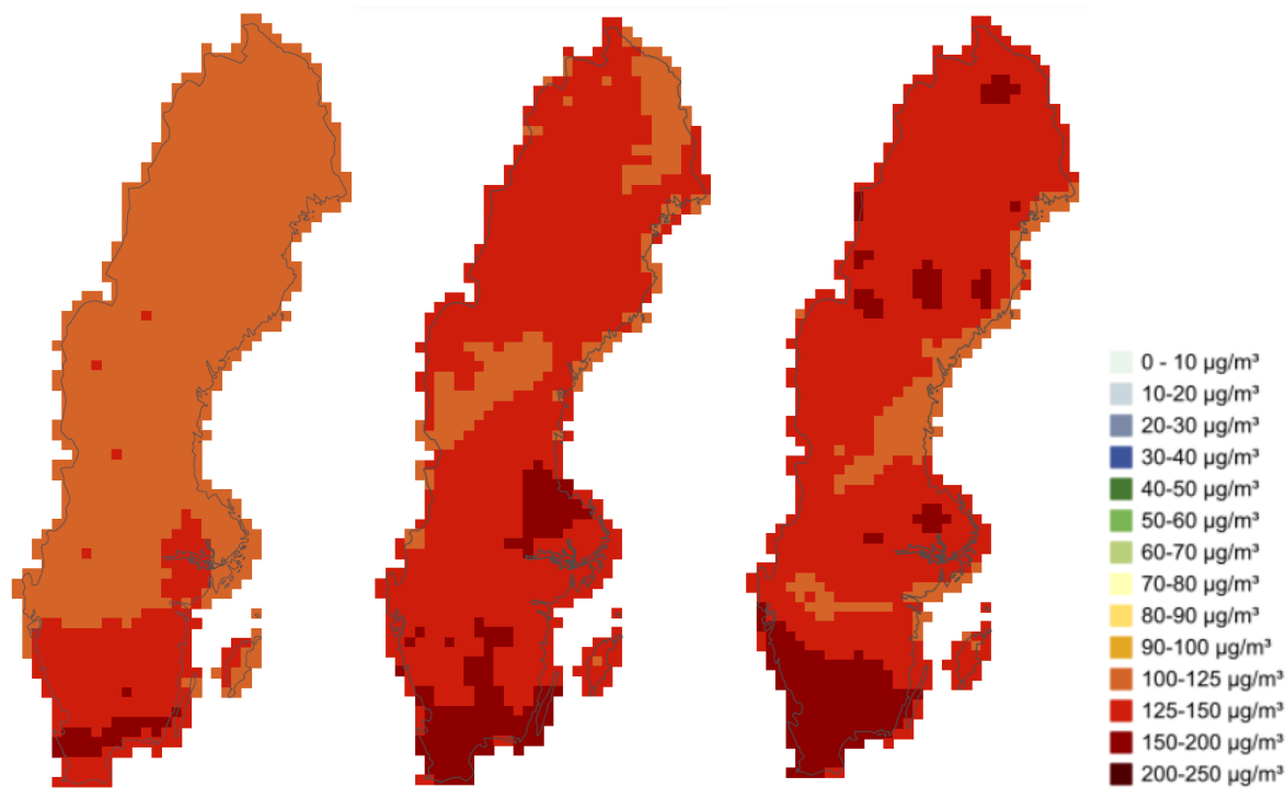
Figur 26. Årets maximala entimmesmedelvärde år 2017 (vänster), 2018 (mitten) och 2019 (höger) för halt i luft av marknära ozon.
