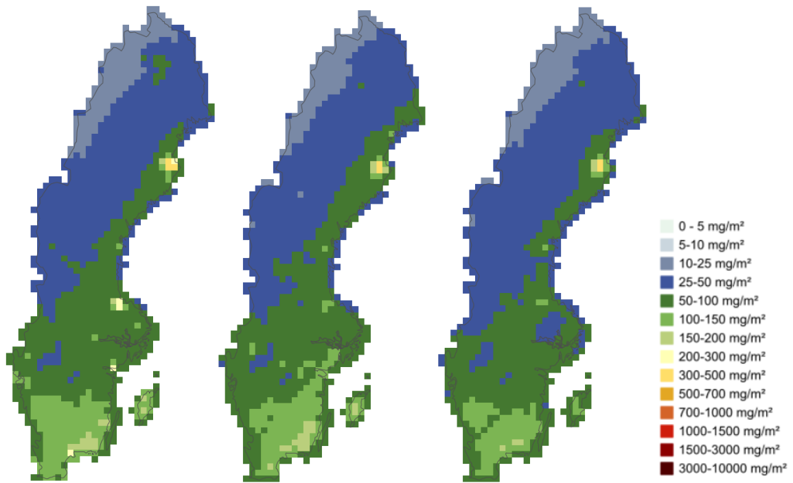
Figur 19. Torrdeposition av oxiderat svavel utan havssalt för år 2017 (vänster), 2018 (mitten) och 2019 (höger). Enhet: mg S m -2 .
