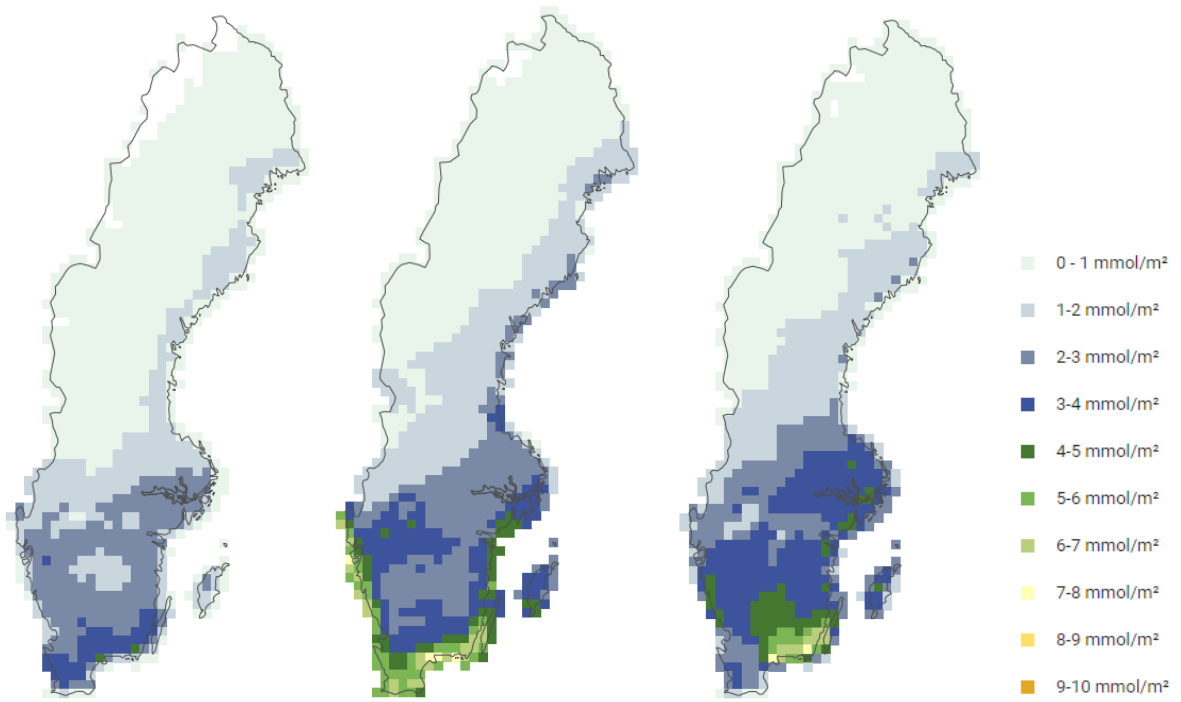
Figur 36. POD6 för potatis under 2017 (vänster), 2018 (mitten) och 2019 (höger).
