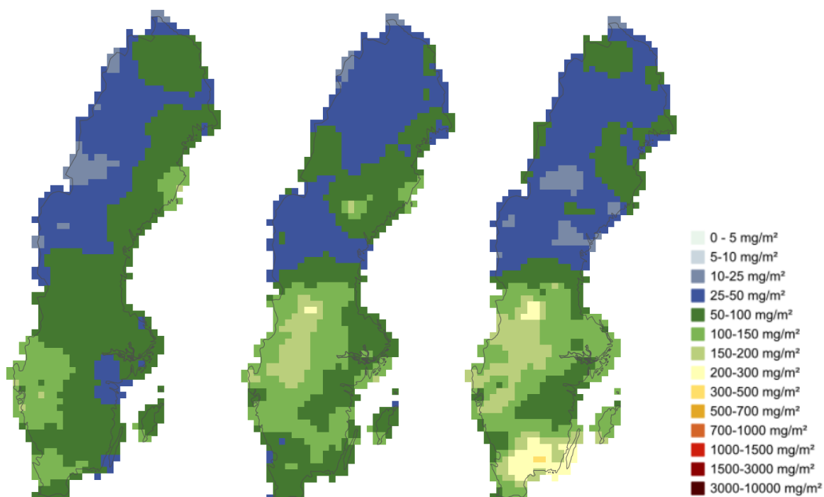
Figur 18. Våtdeposition av oxiderat svavel utan havssalt för år 2017 (vänster), 2018 (mitten) och 2019 (höger). Enhet: \text{mg S m}^{-2} .
