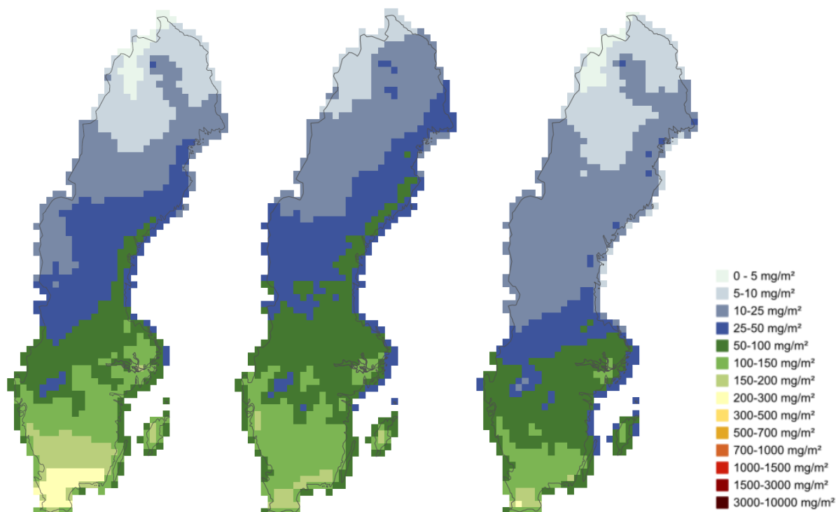
Figur 11. Torrdeposition av oxiderat kväve för år 2017 (vänster), 2018 (mitten) och 2019 (höger). Enhet: \text{mg N m}^{-2} .
