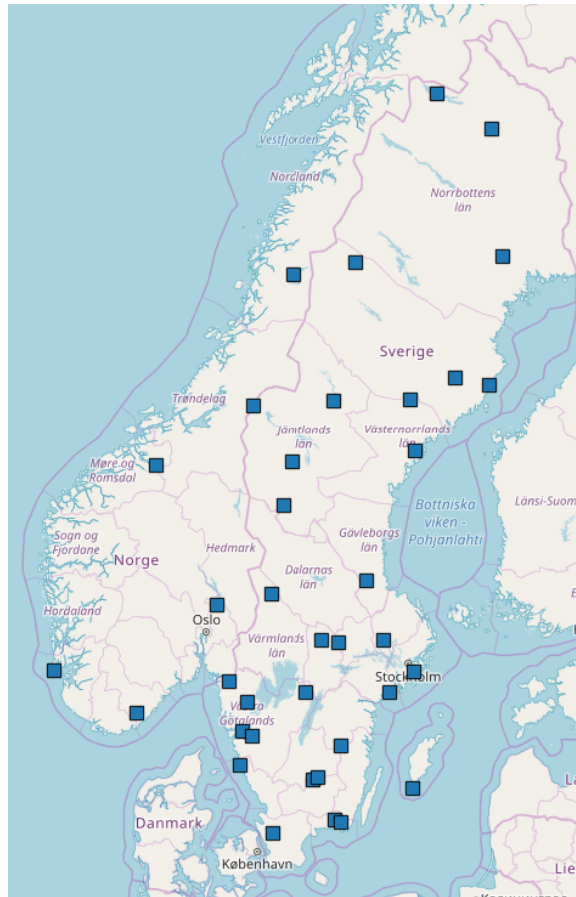
Figur 2. De mätstationer som använts i MATCH Sverigesystemet.
