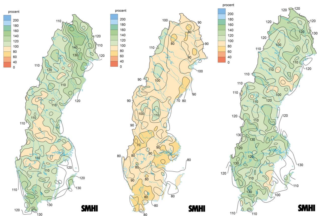
Figur 4. Årsnederbörd (i procent) av den normala årsnederbörden (medelvärde 1961-1990) för år 2017 (vänster), 2018 (mitten) och 2019 (höger). ( https://www.smhi.se/data/meteorologi/kartor/arsnederbord-procent-av-normal )
