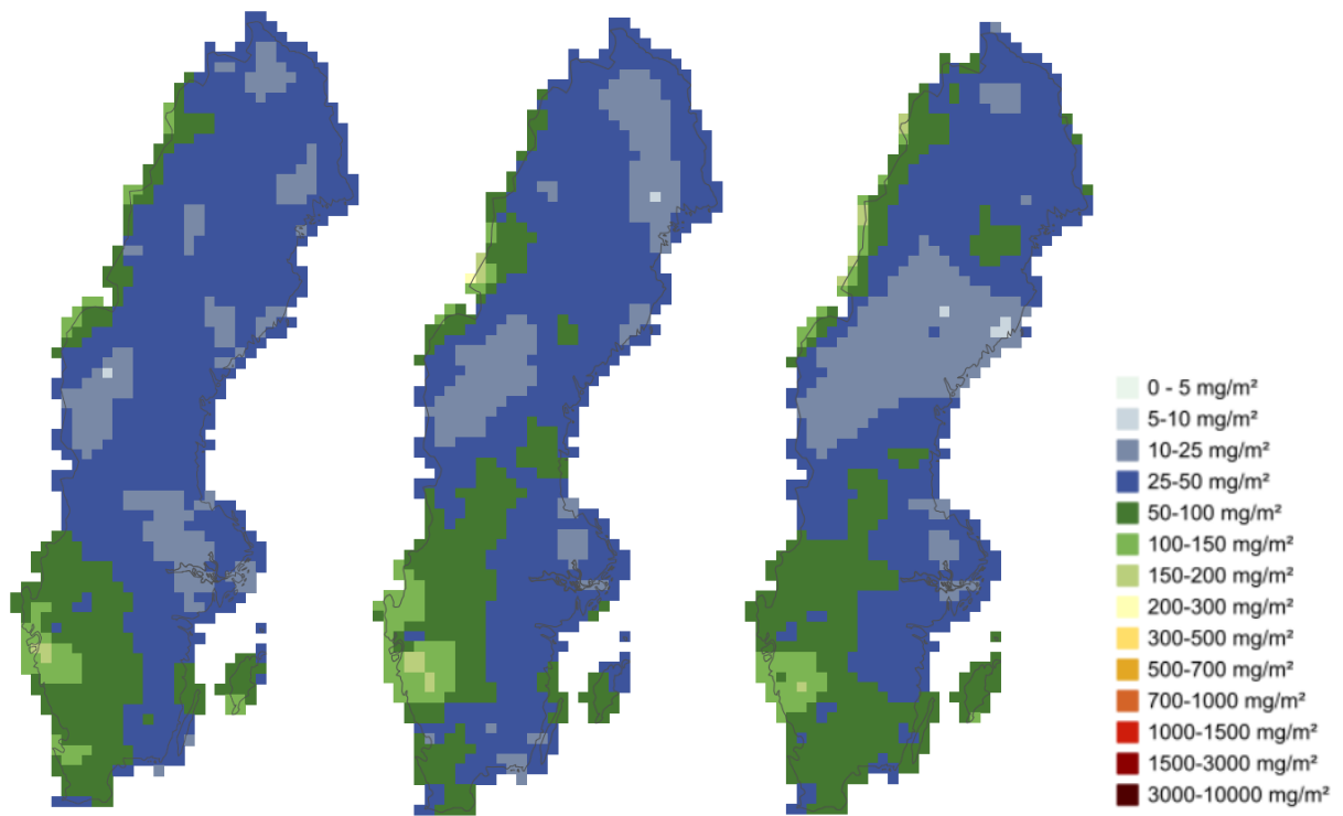
Figur 24. Våtdeposition av magnesium år 2017 (vänster), 2018 (mitten) och 2019 (höger). Enhet: mg Mg m -2 .
