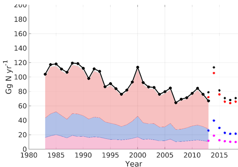
Figur 13. Total deposition av reducerat kväve till Sverige under perioden 1983-2019 (svart), och bidrag till depositionen till skogar (röd), vattenytor (blå) och jordbruksmark (rosa). Ackumulerad deposition av bidragen visas som ytor och cirklar. Total deposition (svart) innehåller utöver dessa bidrag även deposition till övriga ytor, t.ex. urban miljö. Linjer/ytor återanalyserade depositionen med MATCH Sverigesystemet 1983-2013. Cirklar deposition enligt operationella MATCH Sverigesystemets skattning 2013-2019. Skillnader 2013 härleddes till olika indata och mängd av mätdata, se Andersson et al., 2018.
