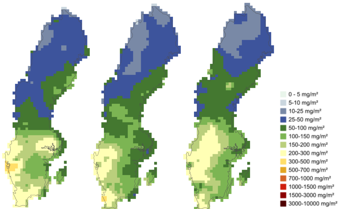
Figur 14. Våtdeposition av reducerat kväve för år 2017 (vänster), 2018 (mitten) och 2019 (höger). Enhet: \text{mg N m}^{-2} .
