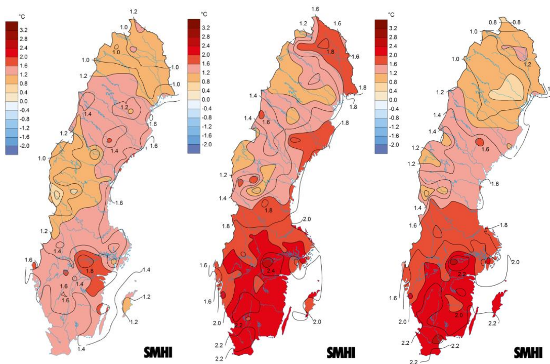
Figur 3. Årsmedeltemperaturens avvikelse (i °C) från den normala årsmedeltemperaturen (medelvärde 1961-1990) för år 2017 (vänster), 2018 (mitten) och 2019 (höger). ( https://www.smhi.se/data/meteorologi/kartor/arsmedeltemperatur-avvikelse )
