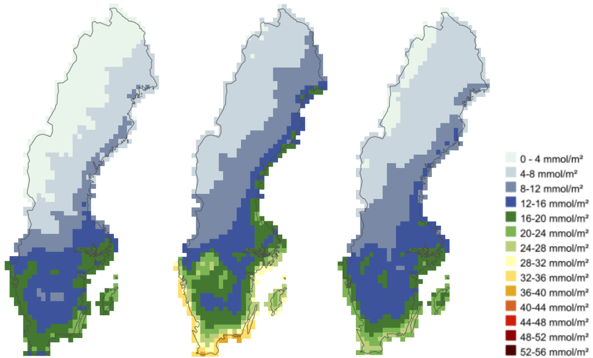
Figur 32. POD3 för generisk gräs under 2017 (vänster), 2018 (mitten) och 2019 (höger).
