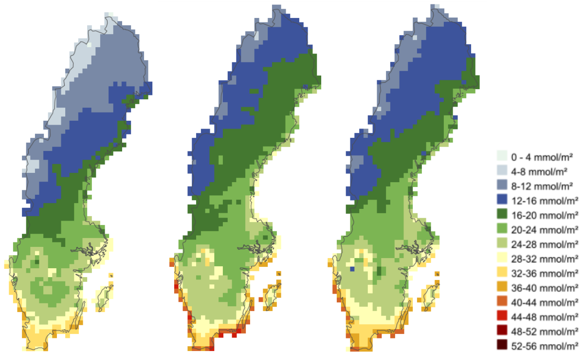
Figur 34. POD1 för björk under 2017 (vänster), 2018 (mitten) och 2019 (höger).
