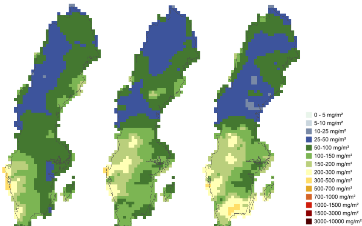
Figur 21. Våtdeposition av oxiderat svavel inklusive havssalt för år 2017 (vänster), 2018 (mitten) och 2019 (höger). Enhet: mg S m -2 .
