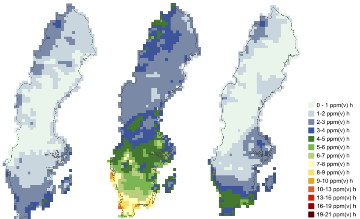
Figur 30. AOT40 för grödor år 2017 (vänster), 2018 (mitten) och 2019 (höger).
