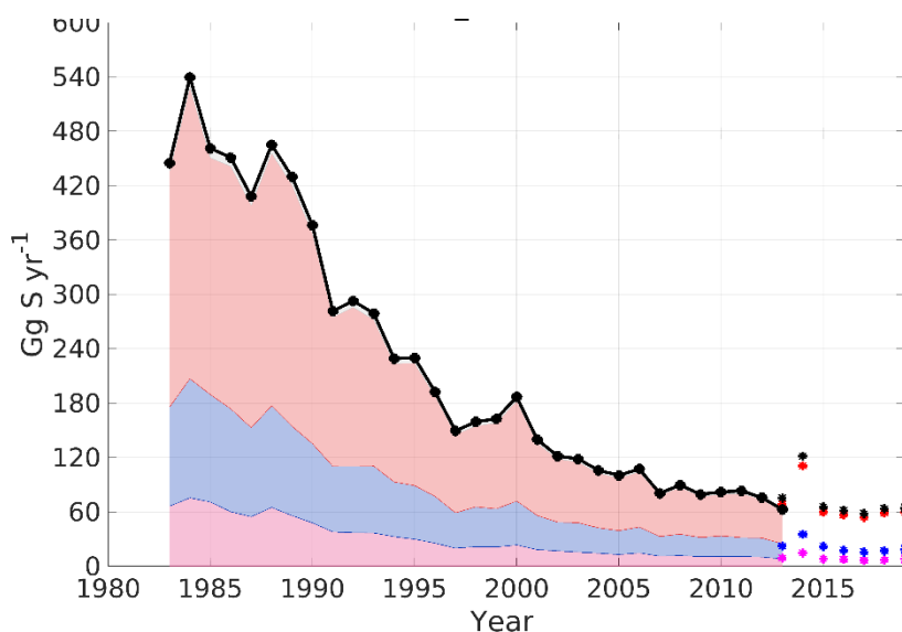
Figur 17. Total deposition av oxiderat svavel utan havssaltsbidrag till Sverige under perioden 1983-2019 (svart), och bidrag till depositionen till skogar (röd), vattenytor (blå) och jordbruksmark (rosa). Ackumulerad deposition av bidragen visas som ytor och cirklar. Total deposition (svart) innehåller utöver dessa bidrag även deposition till övriga ytor, t.ex. urban miljö. Linjer/ytor återanalyserade depositionen med MATCH Sverigesystemet 1983-2013. Cirklar deposition enligt operationella MATCH Sverigesystemets skattning 2013-2019. Skillnader 2013 härleddes till olika indata och mängd av mätdata, se Andersson et al., 2018.
