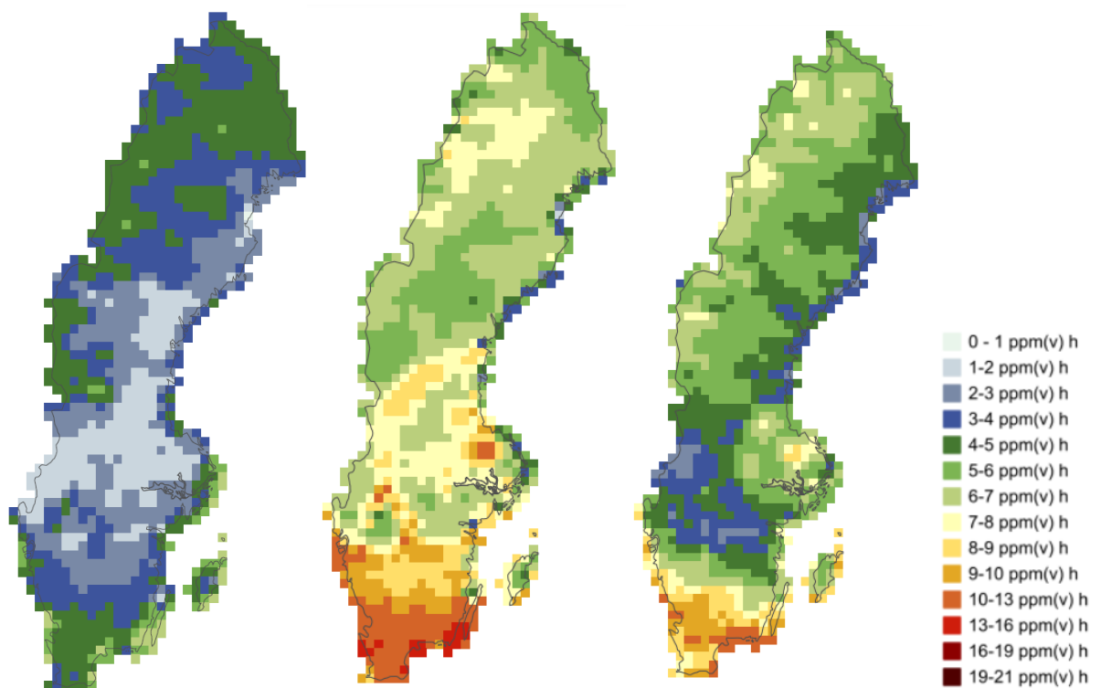
Figur 31. AOT40 för skog år 2017 (vänster), 2018 (mitten) och 2019 (höger).
