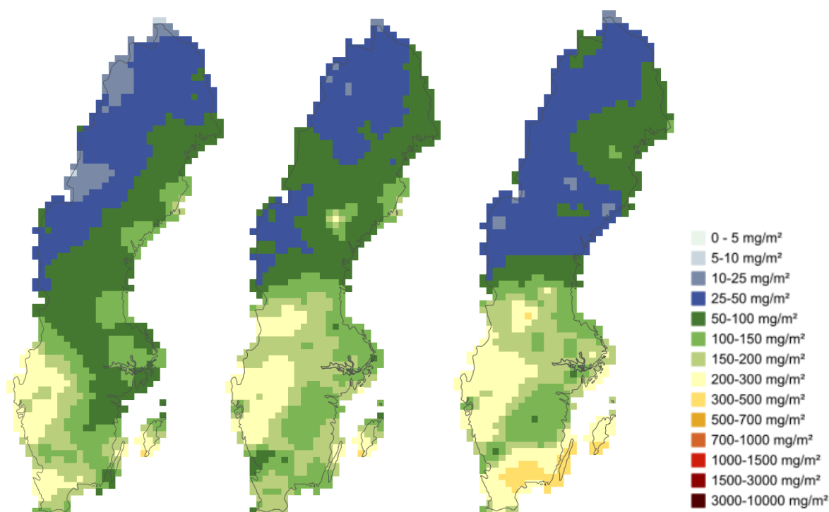
Figur 10. Våtdeposition av oxiderat kväve för år 2017 (vänster), 2018 (mitten) och 2019 (höger). Enhet: \text{mg N m}^{-2} .
