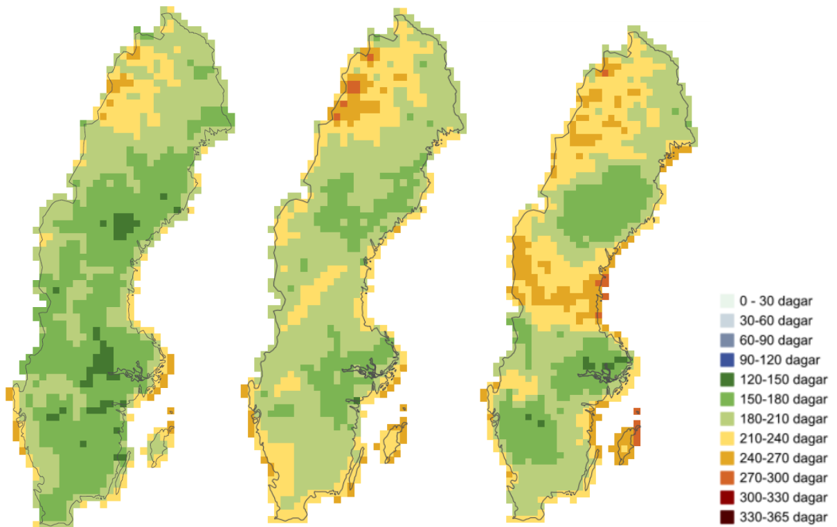
Figur 28. Antal dagar då halt i luft av marknära ozon överstiger 70 \mu\text{g}/\text{m}^3 år 2017 (vänster), 2018 (mitten) och 2019 (höger).
