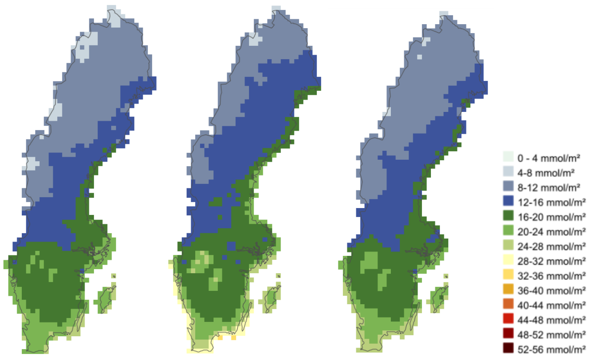
Figur 33. POD1 för generisk lövskog under 2017 (vänster), 2018 (mitten) och 2019 (höger).
