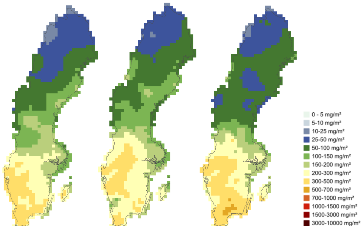
Figur 12. Totaldeposition av reducerat kväve för år 2017 (vänster), 2018 (mitten) och 2019 (höger). Enhet: \text{mg N m}^{-2} .
