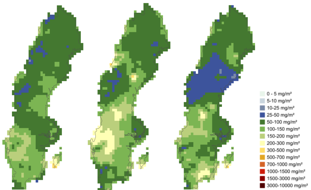
Figur 22. Våtdeposition av kalcium år 2017 (vänster), 2018 (mitten) och 2019 (höger). Enhet: mg Ca m -2 .
