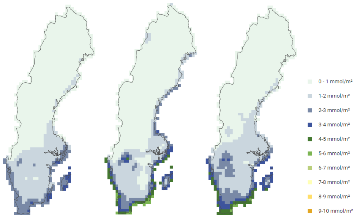
Figur 37. POD6 för vete under 2017 (vänster), 2018 (mitten) och 2019 (höger).
