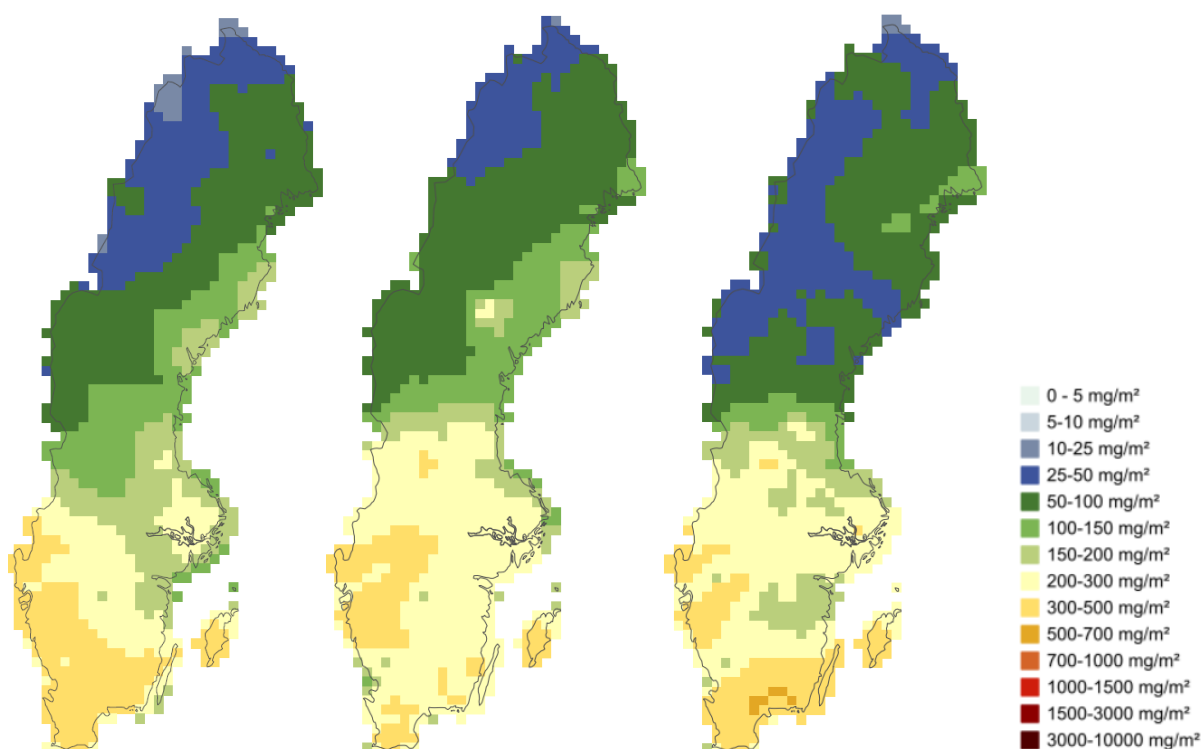
Figur 8. Totaldeposition av oxiderat kväve för år 2017 (vänster), 2018 (mitten) och 2019 (höger). Enhet: mg N m -2 .
