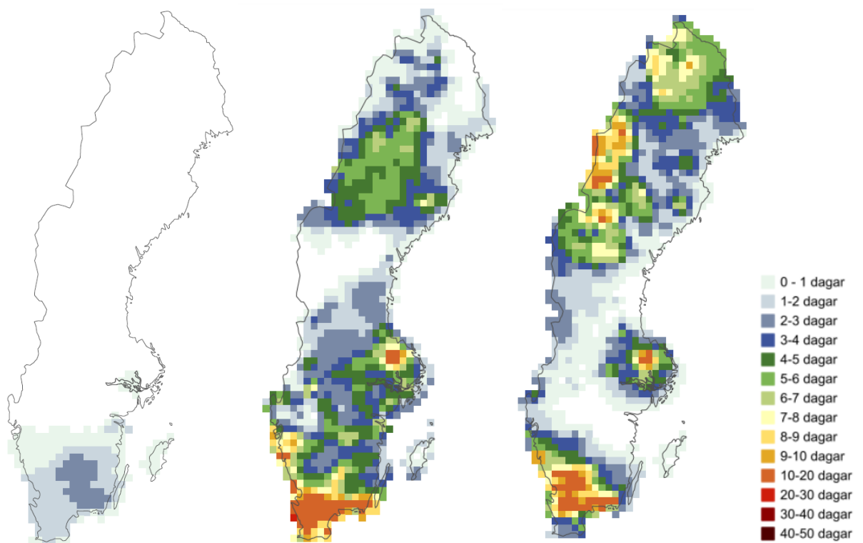
Figur 29. Antal dagar då halt i luft av marknära ozon överstiger 120 \mu\text{g}/\text{m}^3 år 2017 (vänster), 2018 (mitten) och 2019 (höger).
