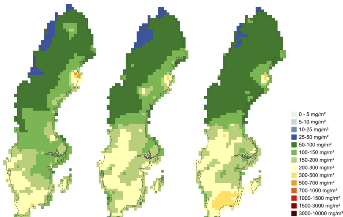
Figur 16. Totaldeposition av oxiderat svavel utan havssalt för år 2017 (vänster), 2018 (mitten) och 2019 (höger). Enhet: mg S m -2 .
