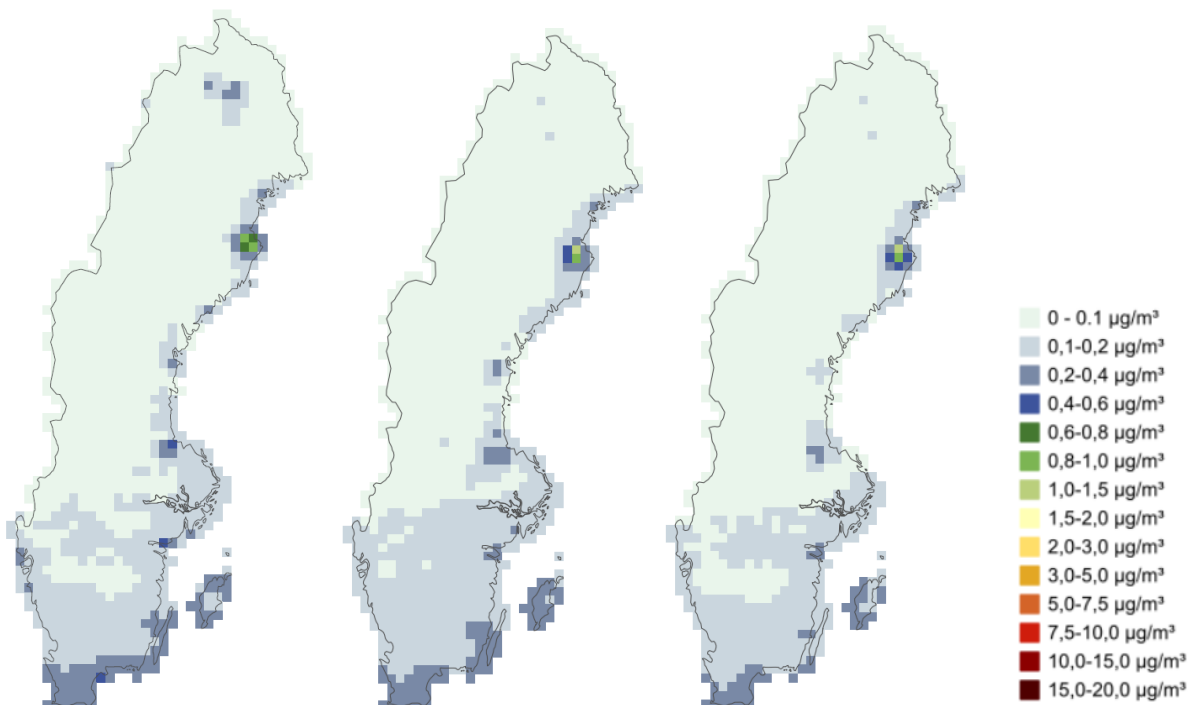
Figur 7. Totala halter av svaveldioxid i luft år 2017 (vänster), 2018 (mitten) och 2019 (höger). Enhet: µg S m -3 .
