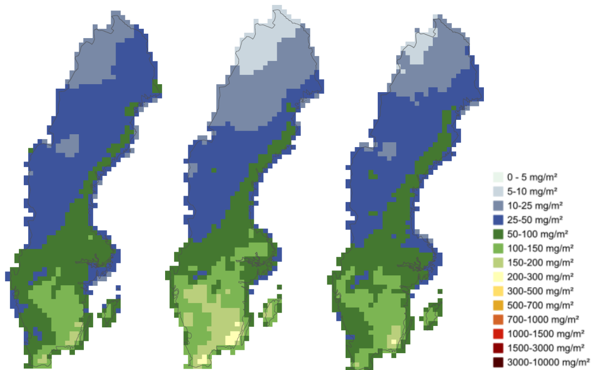
Figur 15. Torrdeposition av reducerat kväve för år 2017 (vänster), 2018 (mitten) och 2019 (höger). Enhet: \text{mg N m}^{-2} .
