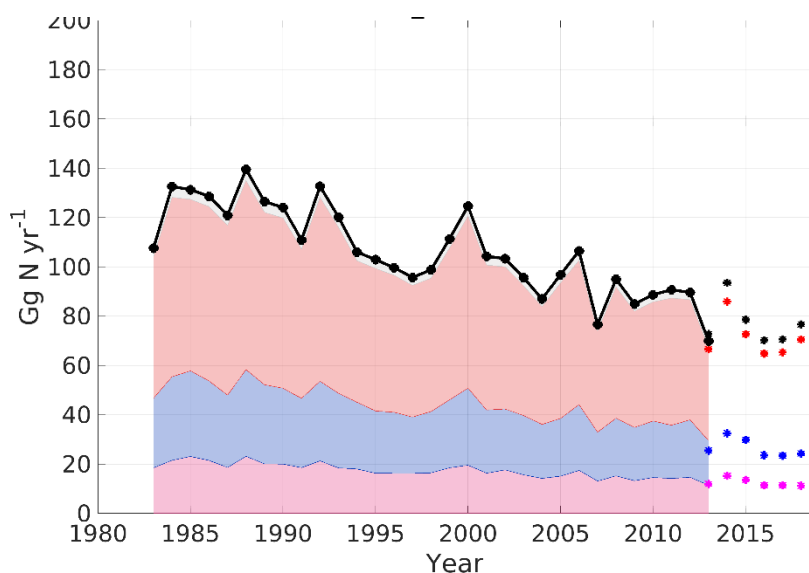
Figur 9. Total deposition av oxiderat kväve till Sverige under perioden 1983-2019 (svart), och bidrag till depositionen till skogar (röd), vattenytor (blå) och jordbruksmark (rosa). Ackumulerad deposition av bidragen visas som ytor och cirklar. Total deposition (svart) innehåller utöver dessa bidrag även deposition till övriga ytor, t.ex. urban miljö. Linjer/ytor återanalyserade depositionen med MATCH Sverigesystemet 1983-2013. Cirklar deposition enligt operationella MATCH Sverigesystemets skattning 2013-2019. Skillnader 2013 härleddes till olika indata och mängd av mätdata, se Andersson et al., 2018.
