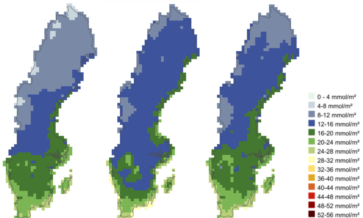
Figur 35. POD1 för gran under 2017 (vänster), 2018 (mitten) och 2019 (höger).
