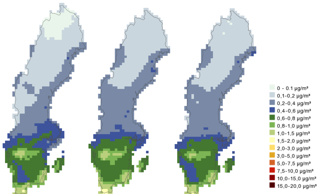
Figur 6. Totala halter av reducerat kväve i luft år 2017 (vänster), 2018 (mitten) och 2019 (höger). Enhet: µg N m -3 .
