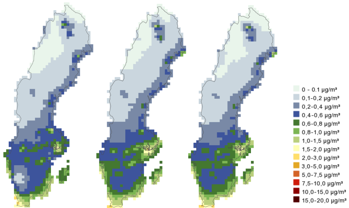
Figur 5. Totala halter av kvävedioxid i luft år 2017 (vänster), 2018 (mitten) och 2019 (höger). Enhet: \mu\text{g N m}^{-3} .
