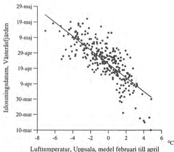
Figur 10. Sambandet mellan islossningsdatum, Västerås fjärd och medeltemperaturen februari till april, Uppsala. 1722-1999.
